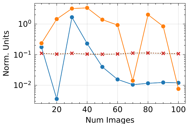
RTE ↓
