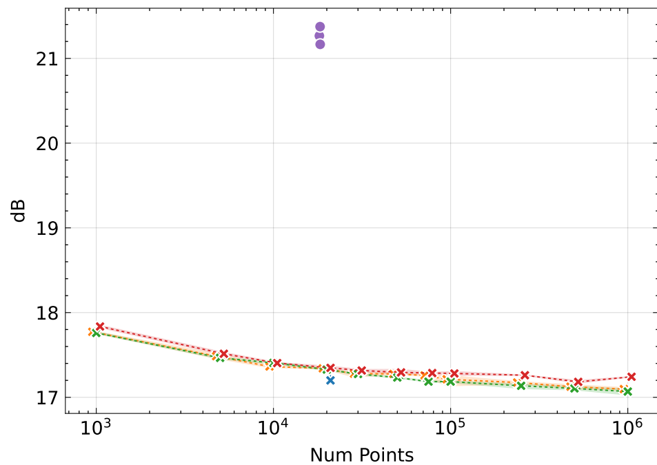
PSNR \uparrow
