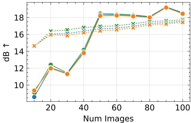
PSNR
