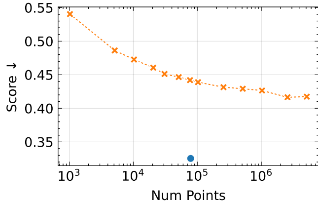
LPIPS
