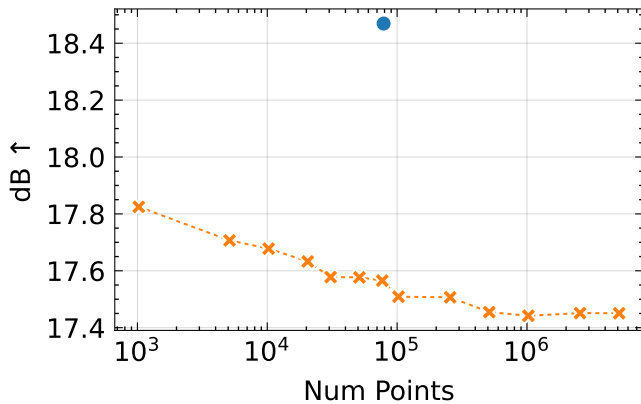
PSNR
