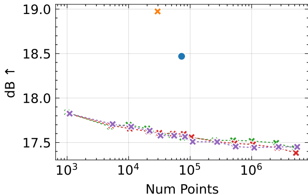
PSNR
