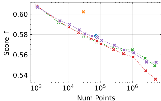
SSIM
