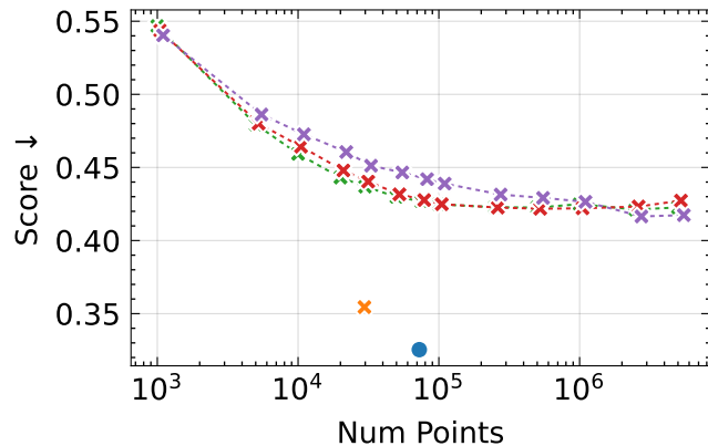
LPIPS
