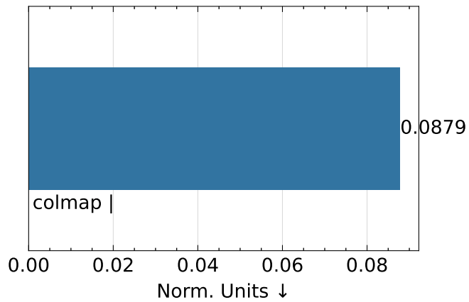
SSIM
