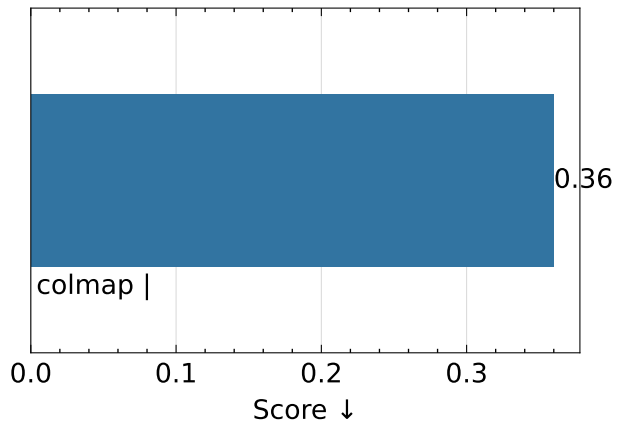
LPIPS
