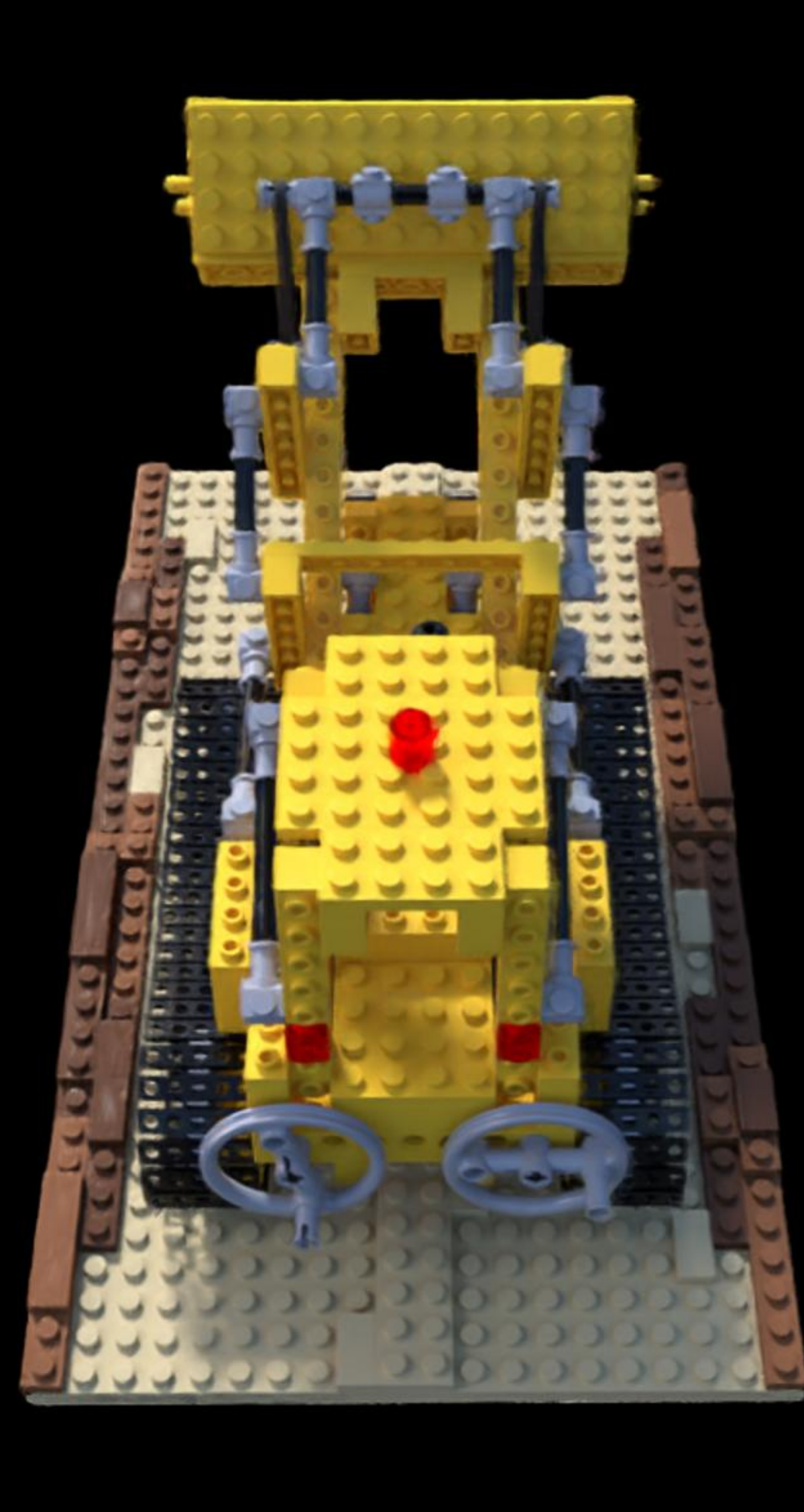
Config: VGGT | num_images=87 PSNR: 20.20 | LPIPS: 0.1058 | SSIM: 0.7610
