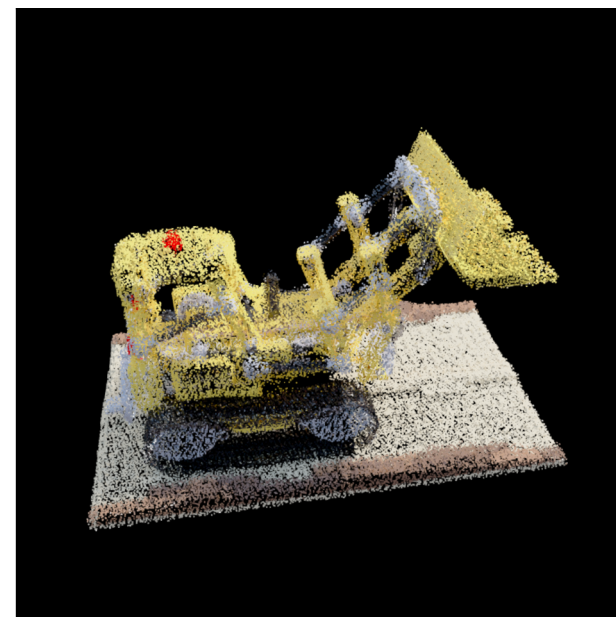
VGGT | voxels | num_points=87000 (Zoom)
