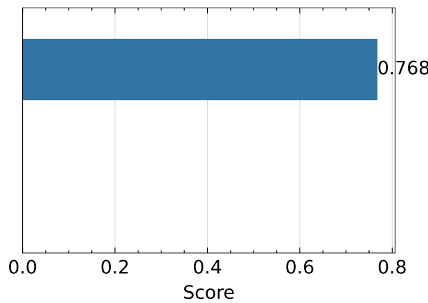
SSIM ↑ - bonsai
