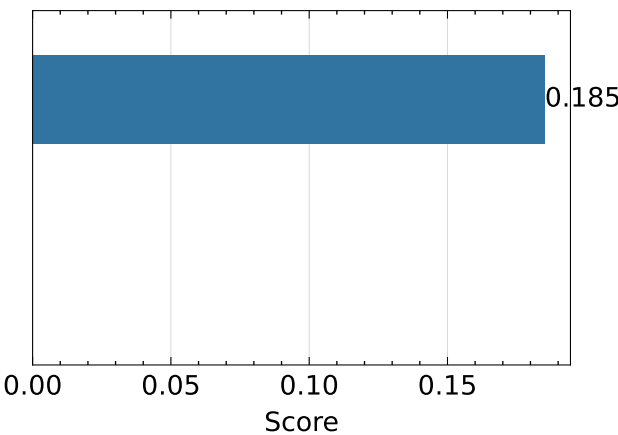
SSIM ↑ - bonsai
