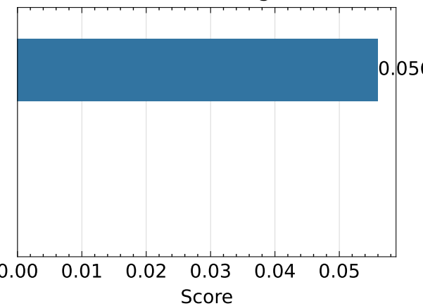
SSIM ↑ - lego
