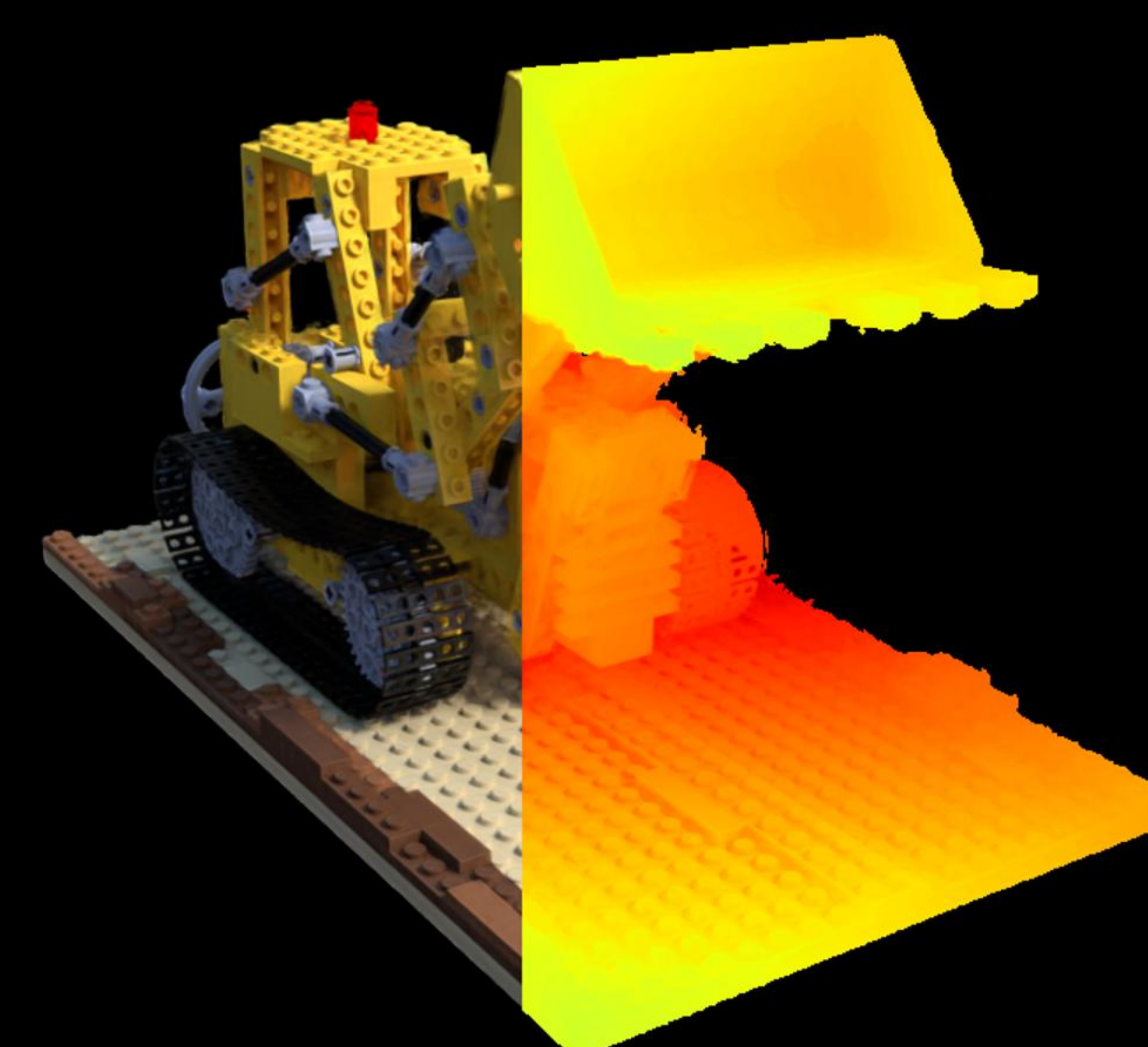
Config: VGGT | PSNR: 18.82 | LPIPS: 0.0814 | SSIM: 0.7420
