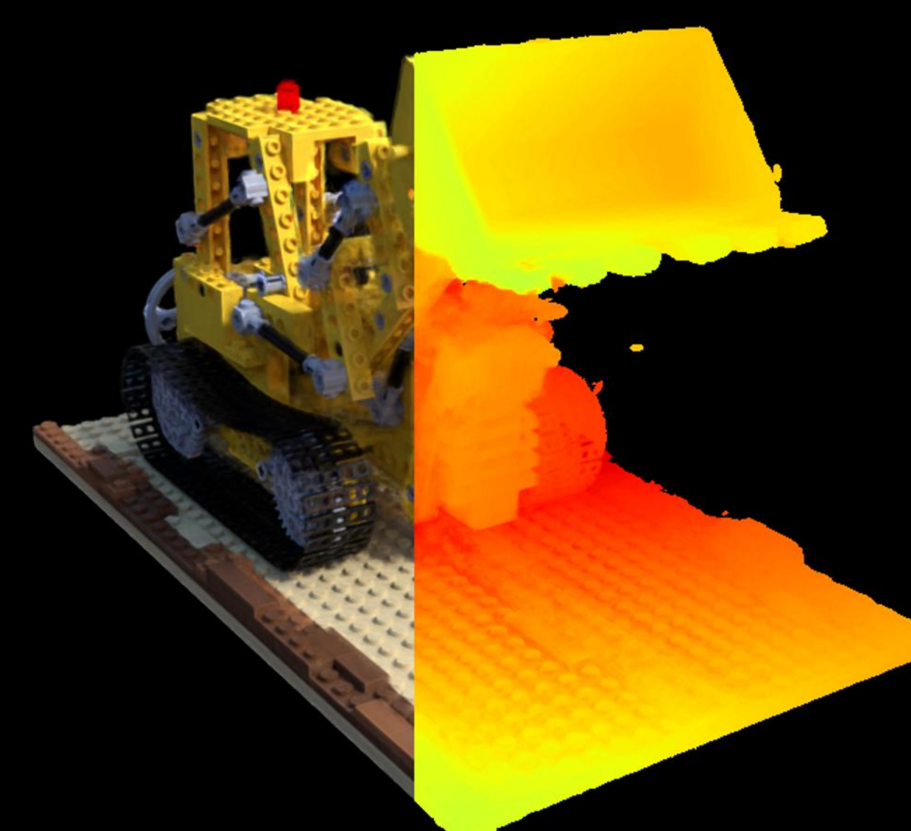
Config: VGGT | standard PSNR: 18.92 | LPIPS: 0.0888 | SSIM: 0.7430
