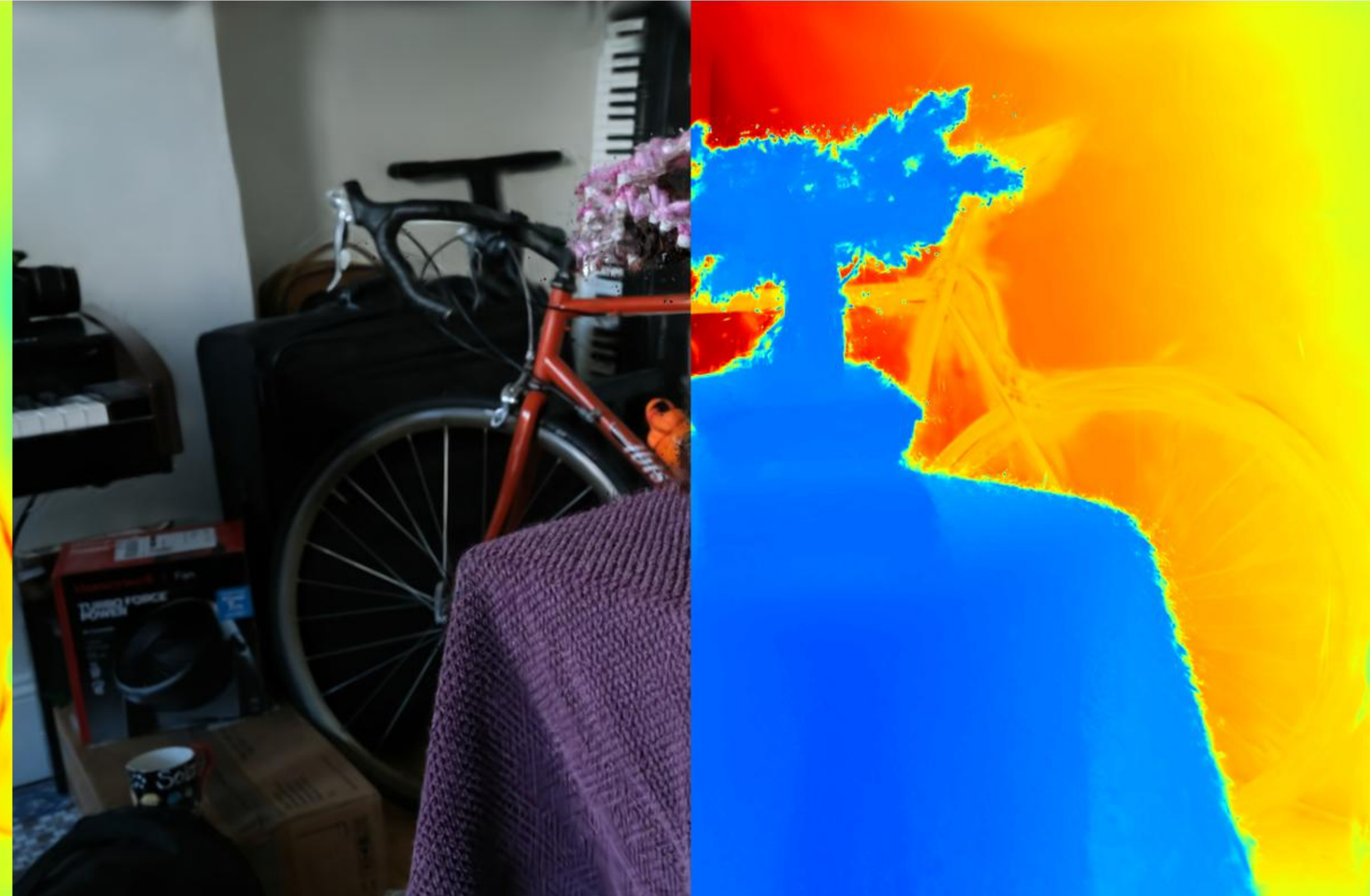
Config: VGGT | | points | depth_lambda=1.0 PSNR: 17.53 | LPIPS: 0.3273 | SSIM: 0.5641
