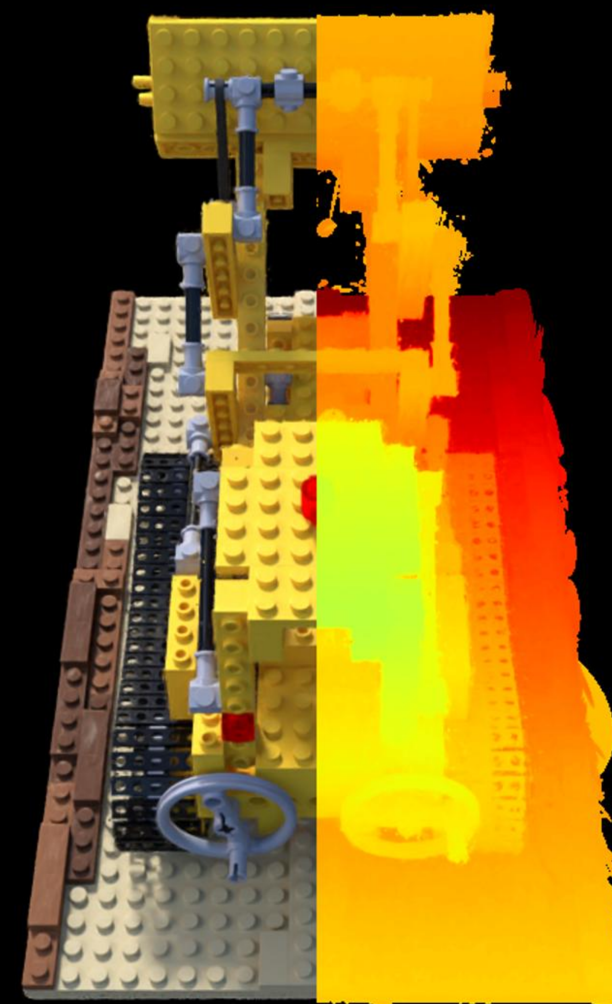
Config: VGGT | | points | depth_lambda=1.0 PSNR: 25.94 | LPIPS: 0.0490 | SSIM: 0.9176
