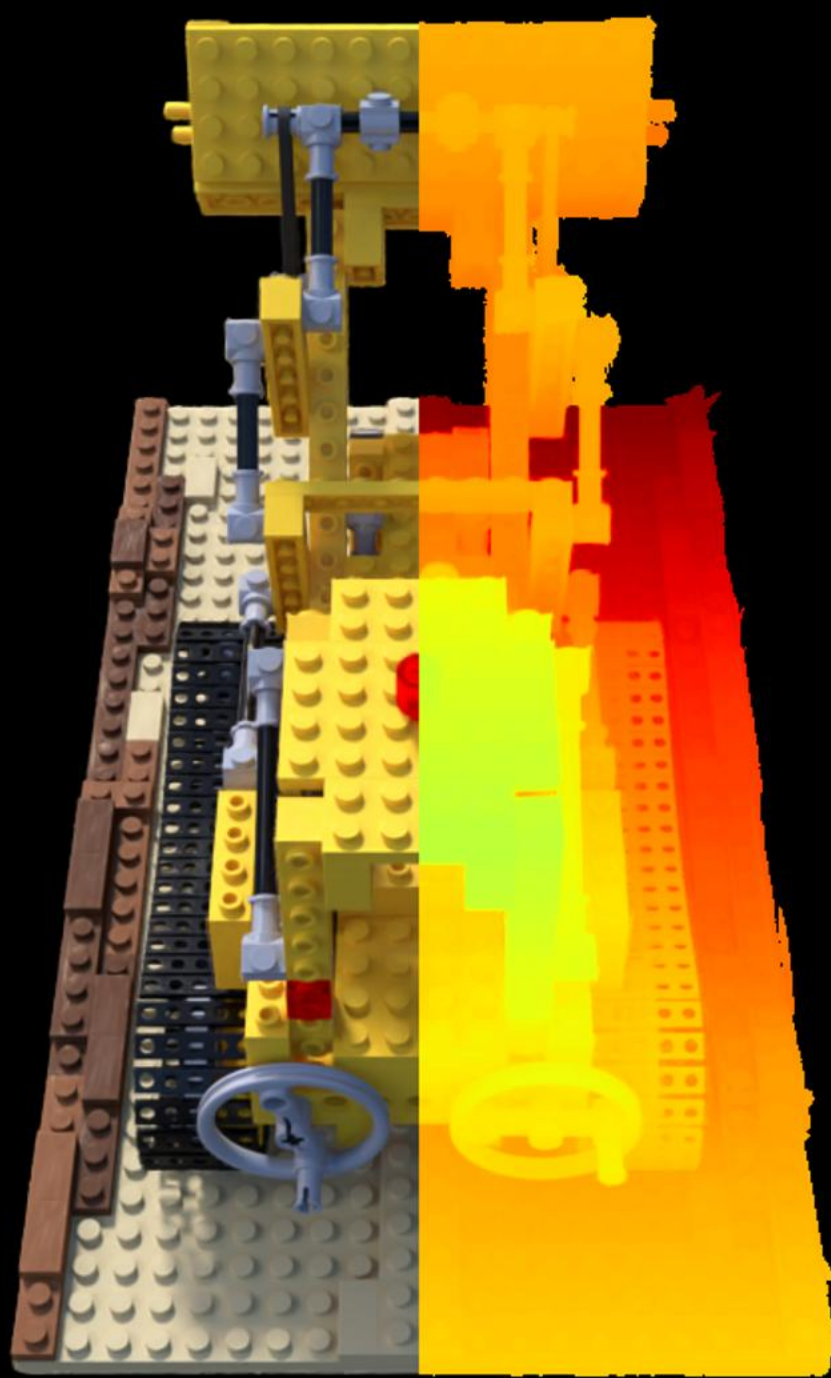
Config: VGGT | | depth_lambda=0.0 PSNR: 25.81 | LPIPS: 0.0485 | SSIM: 0.9226
