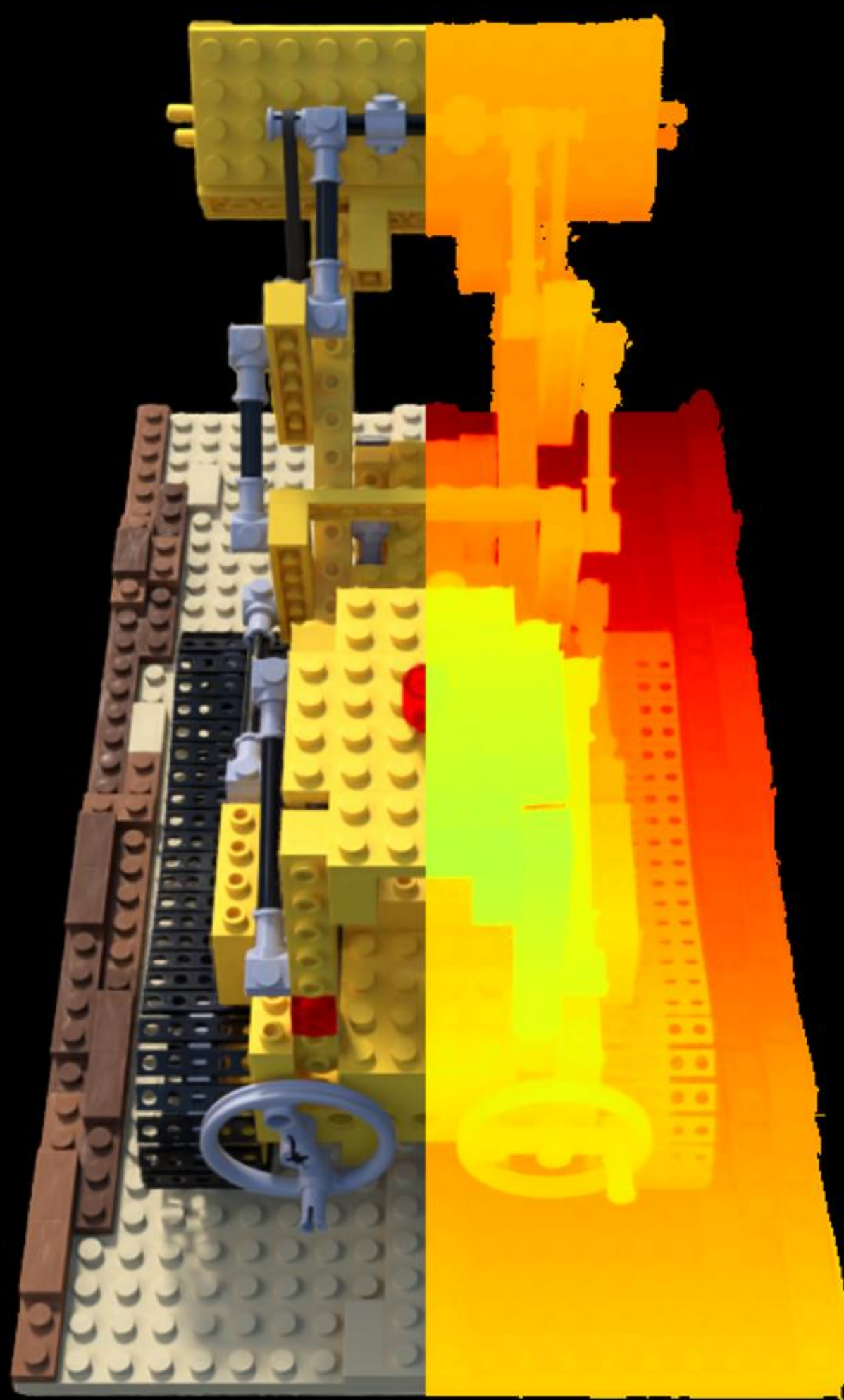
Config: VGGT | | points | depth_lambda=0.01 PSNR: 25.81 | LPIPS: 0.0482 | SSIM: 0.9223
