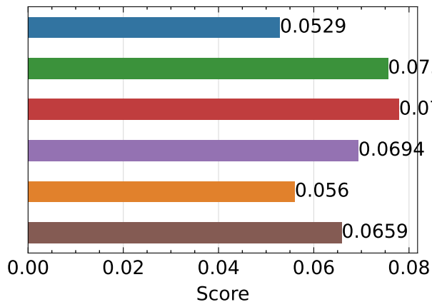
LPIPS ↓
