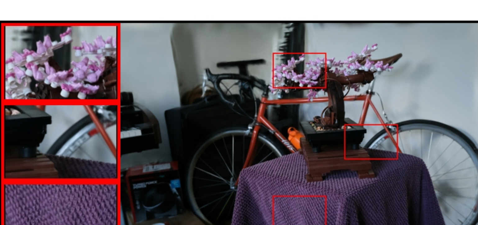
bonsai: VGGT | voxels | num_points=100000 PSNR: 25.99 | LPIPS: 0.2110 | SSIM: 0.8332
