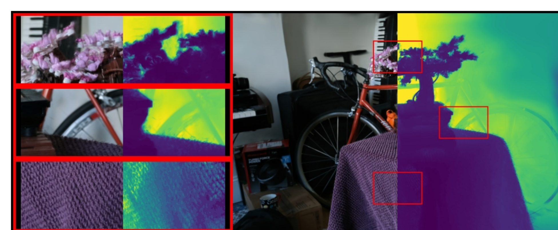
bonsai: VGGT | depth_lambda=0.0 PSNR: 17.42 | LPIPS: 0.3988 | SSIM: 0.5598
