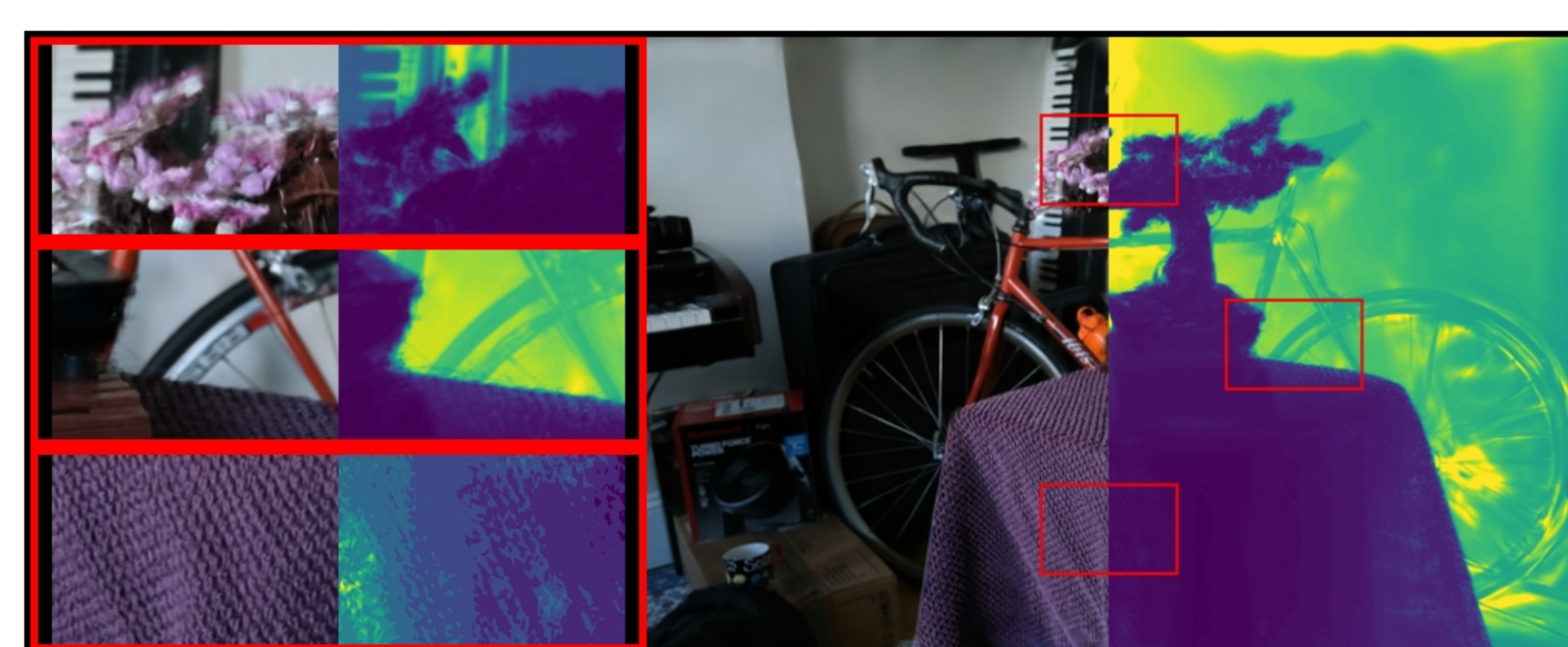
bonsai: VGGT | depth_lambda=10.0 PSNR: 17.76 | LPIPS: 0.3921 | SSIM: 0.5667
