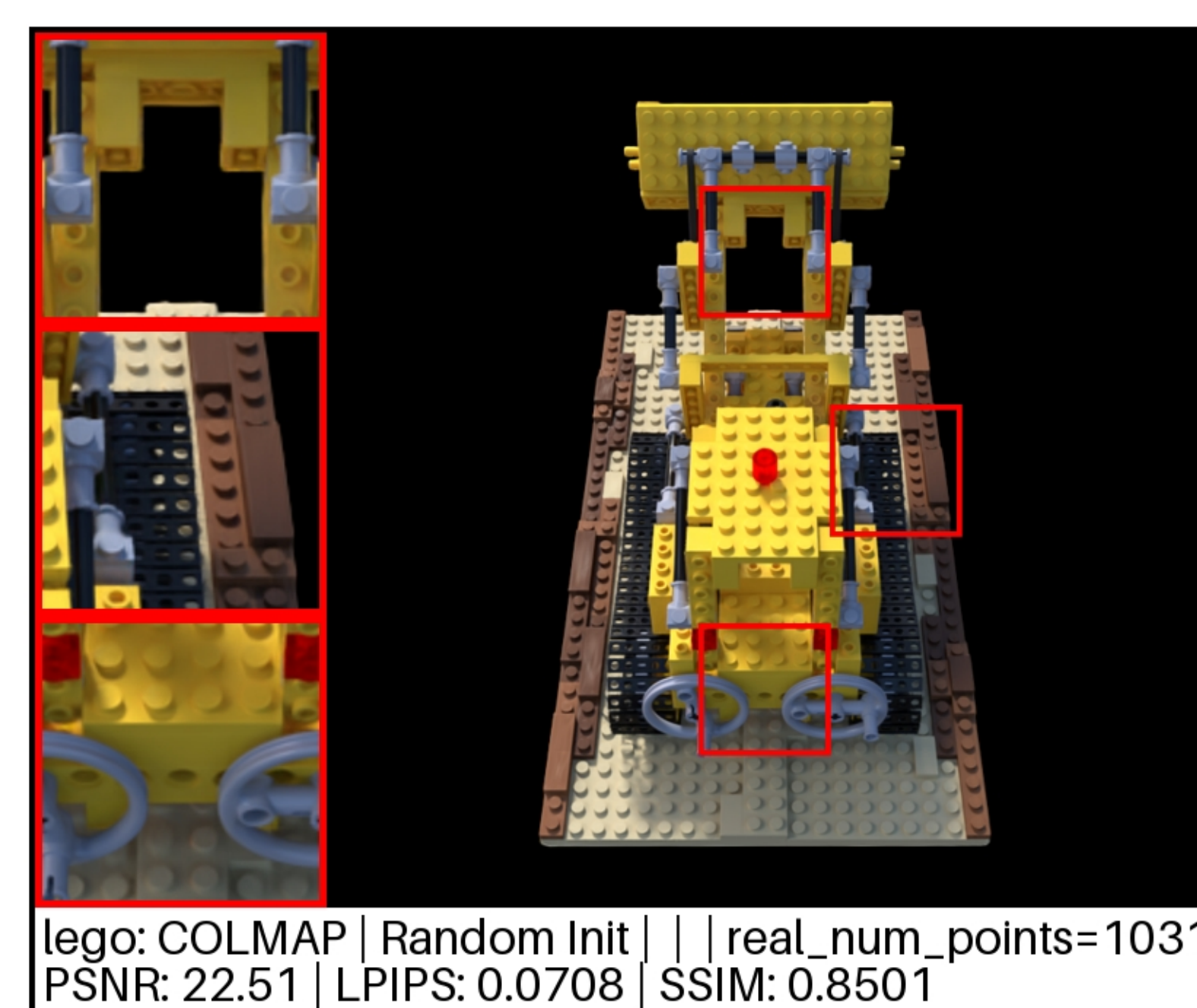
lego: COLMAP | Random Init | | real_num_points=1031 PSNR: 22.51 | LPIPS: 0.0708 | SSIM: 0.8501
