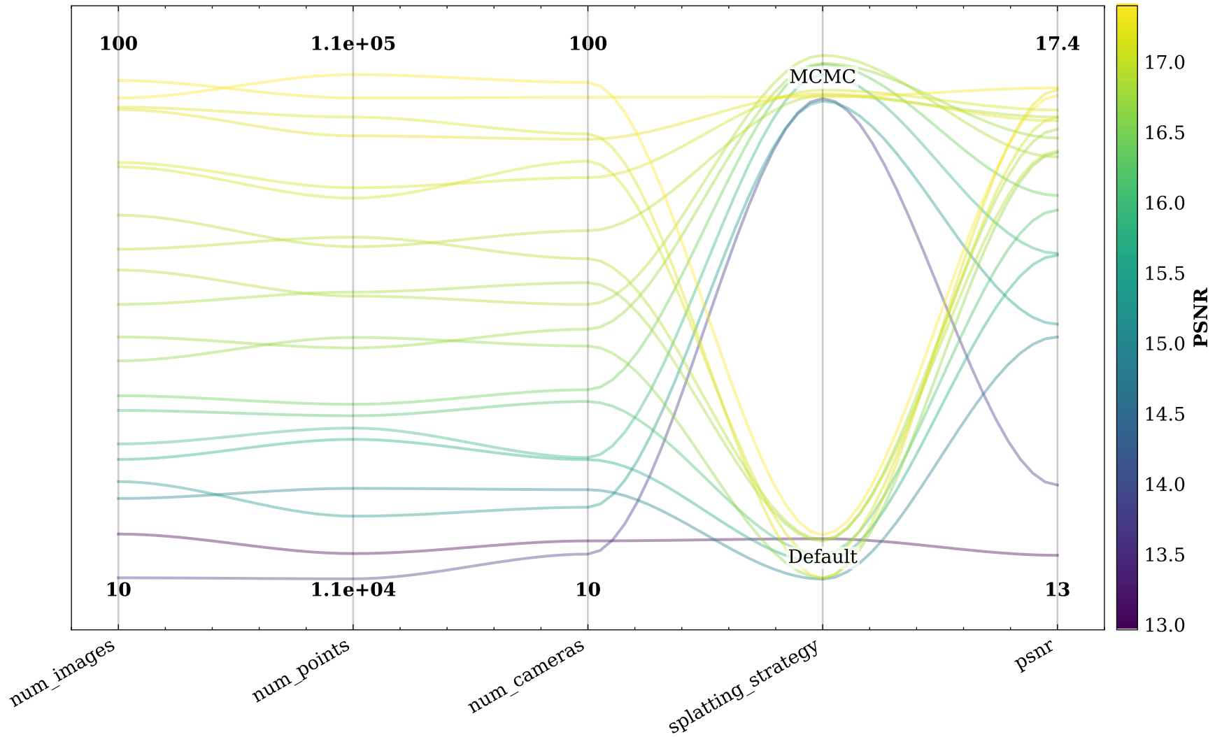
Parallel Coordinate Plot: Parameters vs PSNR
