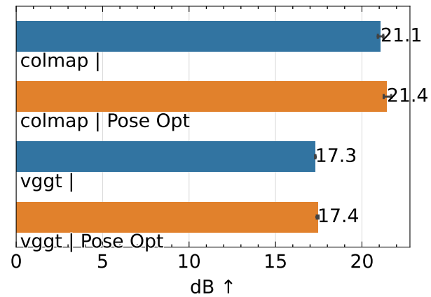
PSNR
