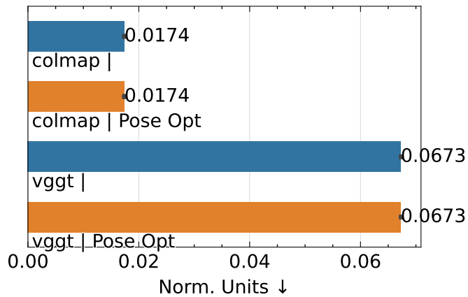
SSIM
