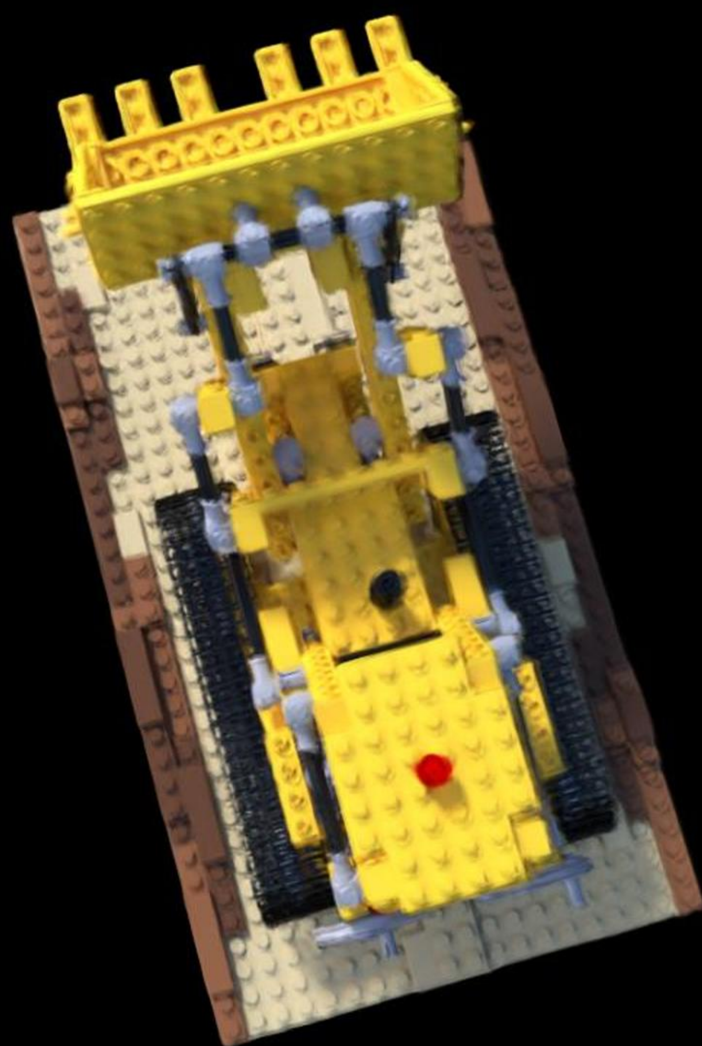
Config: VGGT | num_points=8700 PSNR: 19.10 | LPIPS: 0.1241 | SSIM: 0.7418
