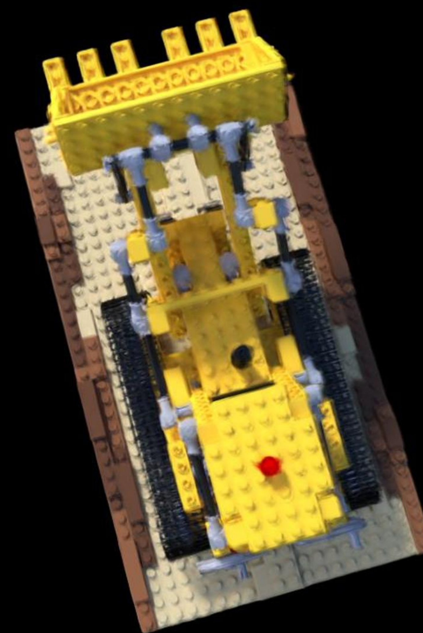
Config: VGGT | num_points=870000 PSNR: 19.24 | LPIPS: 0.1220 | SSIM: 0.7436
