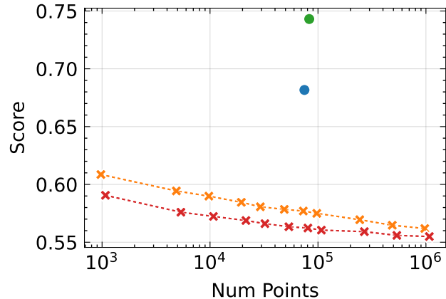
SSIM ↑
