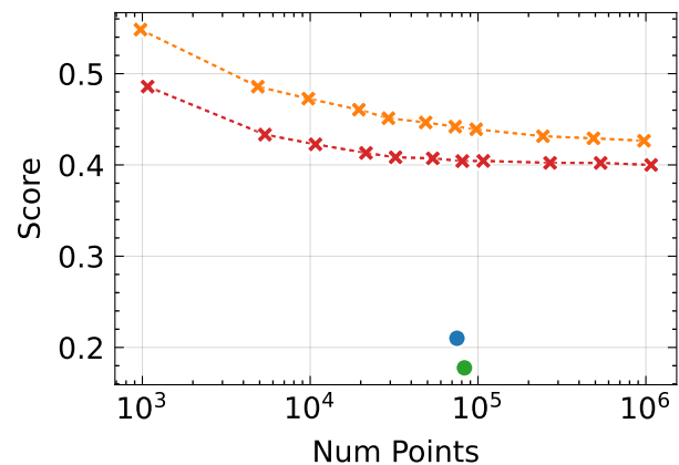
LPIPS ↓
