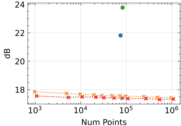
PSNR ↑
