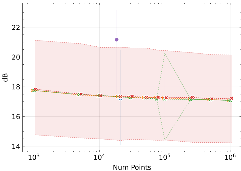
PSNR \uparrow
