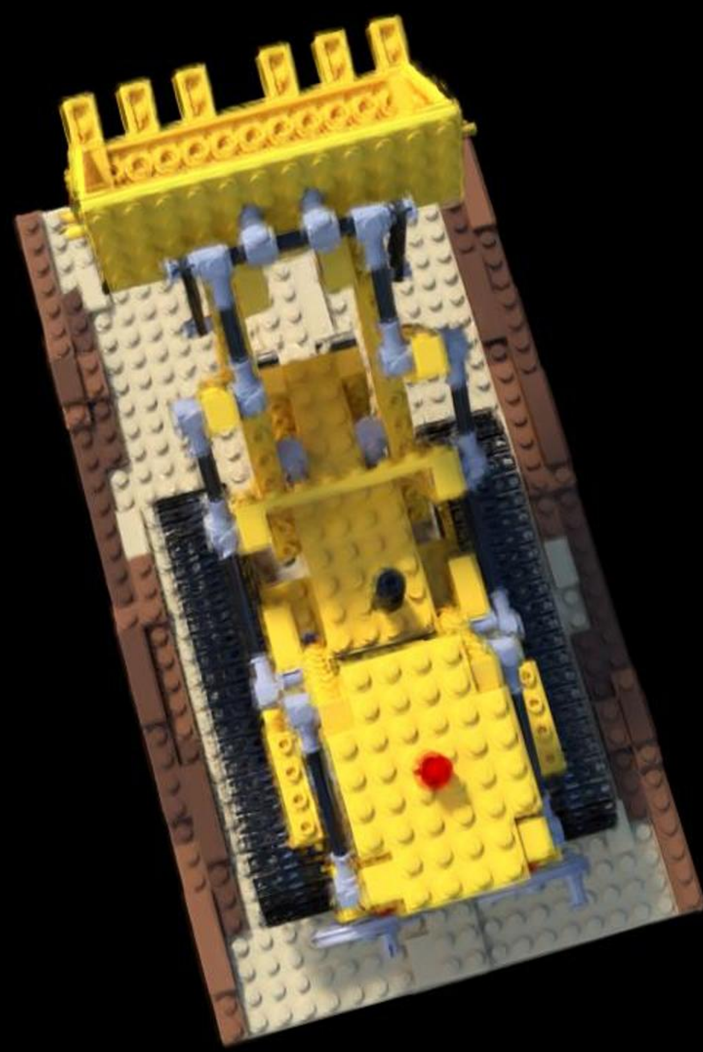
Config: VGGT | ba | num_points=30396 PSNR: 21.91 | LPIPS: 0.0942 | SSIM: 0.8071
