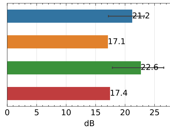
PSNR ↑
