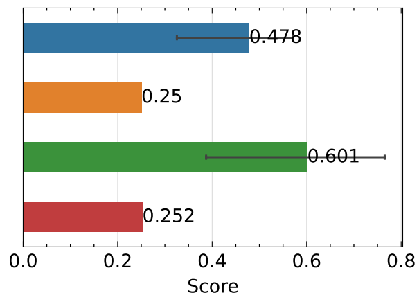
SSIM ↑
