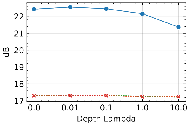
PSNR \uparrow
