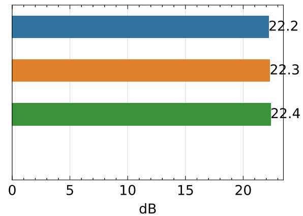
PSNR ↑
