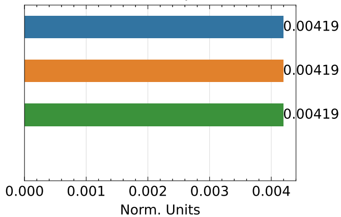
LPIPS ↓
