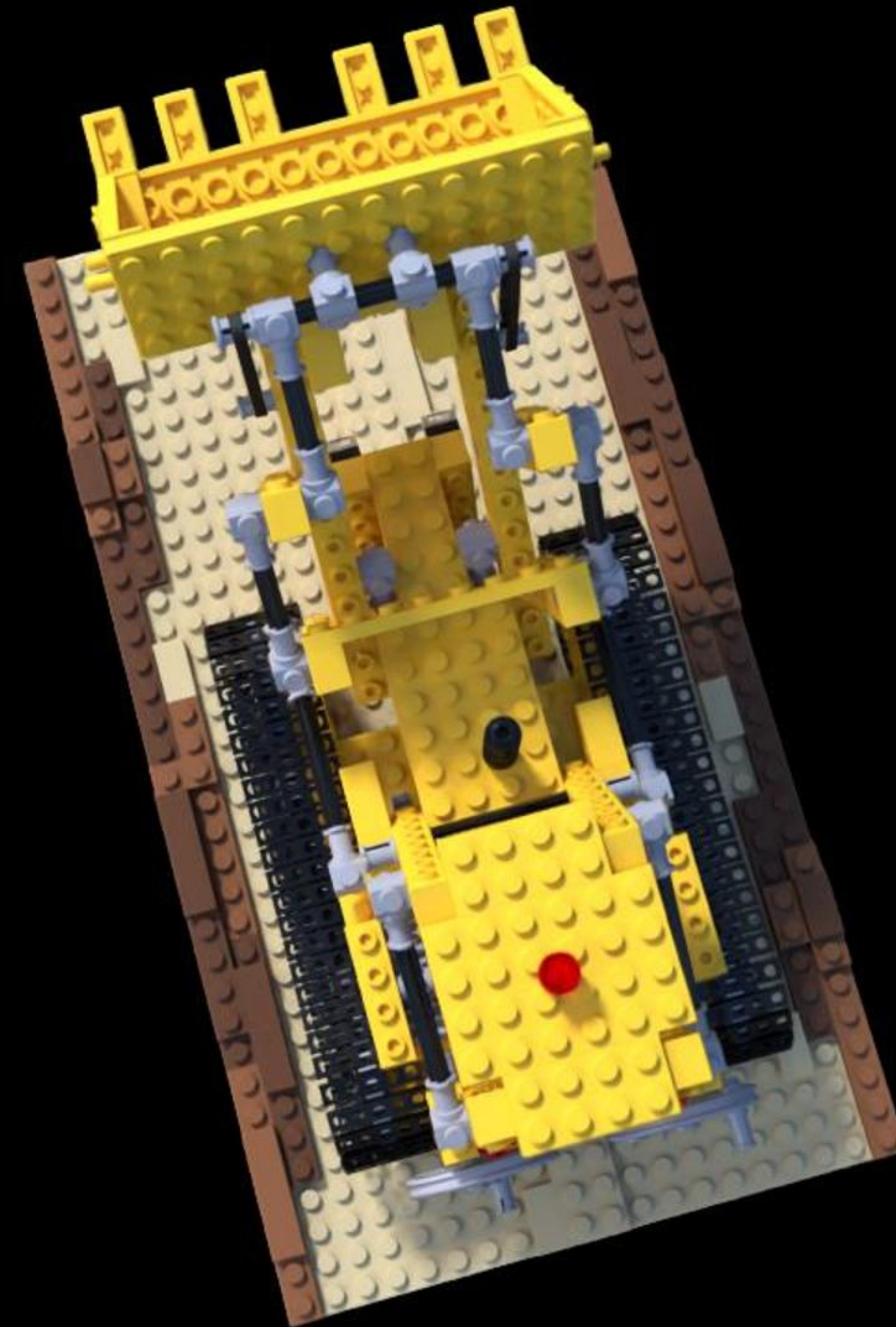
Config: VGGT | | PSNR: 21.11 | LPIPS: 0.0583 | SSIM: 0.8017
