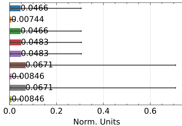
SSIM ↑
