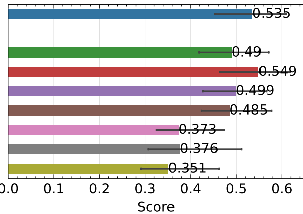
LPIPS ↓
