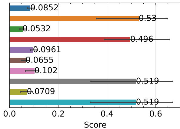
LPIPS ↓
