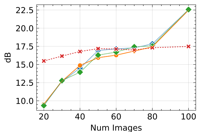
PSNR ↑
