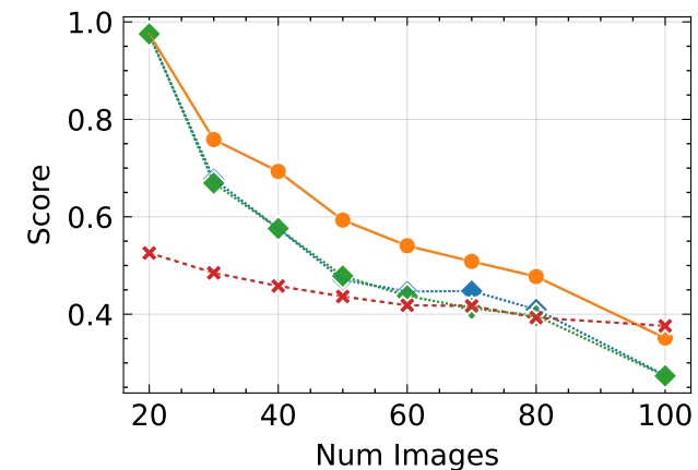
LPIPS ↓
