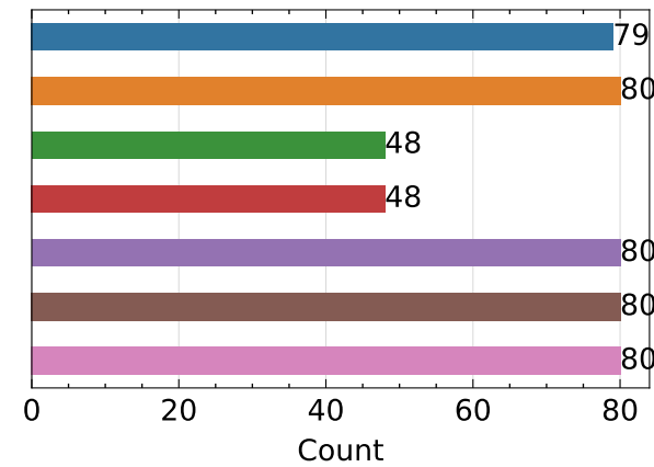
LPIPS ↓
