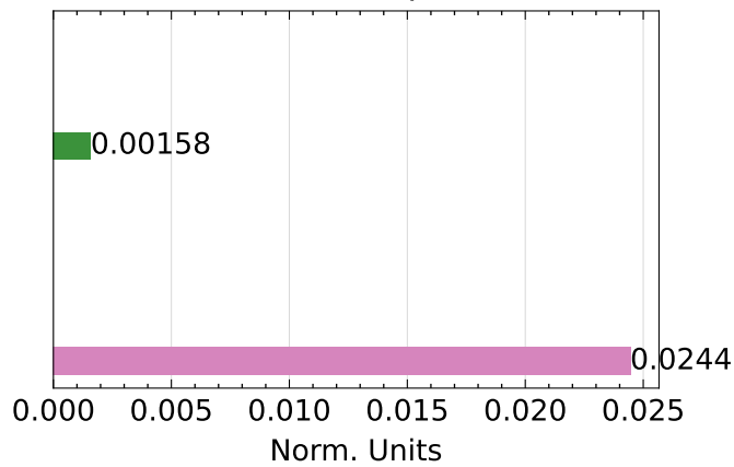
SSIM ↑
