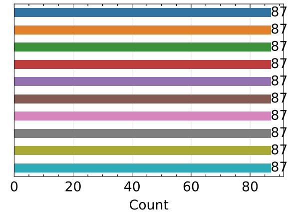
LPIPS ↓
