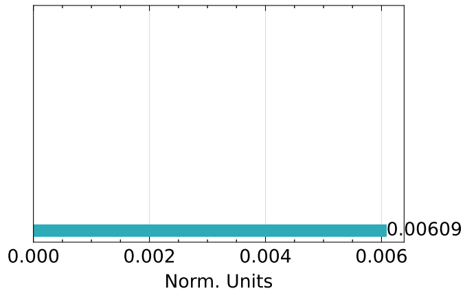
SSIM ↑
