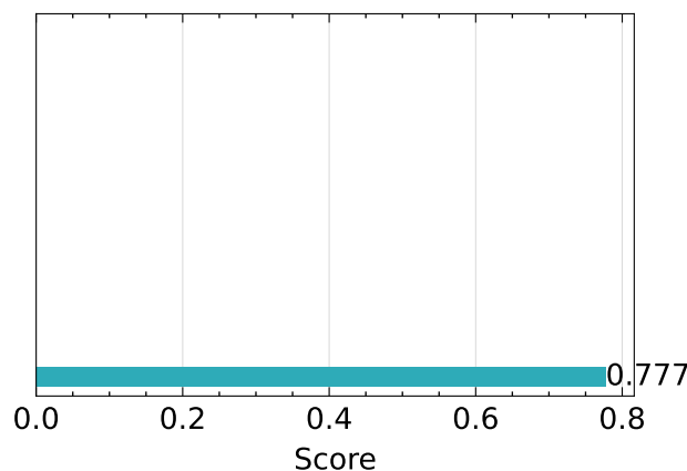
SSIM ↑
