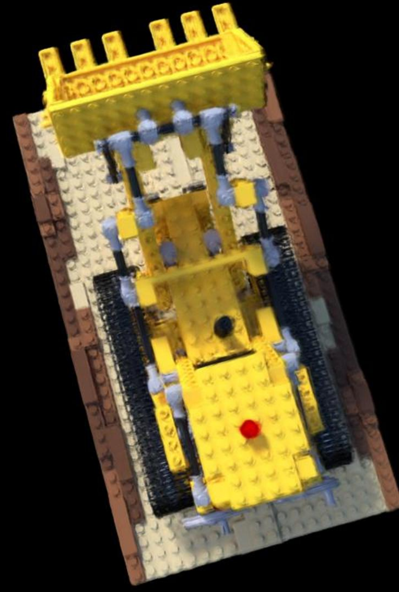
Config: VGGT | 0 | PSNR: 19.12 | LPIPS: 0.1204 | SSIM: 0.7437
