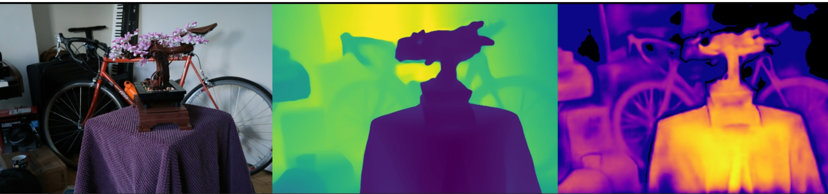
bonsai: VGGT | | Original | Depth (max=2.21) | Confidence (max=5.14)
