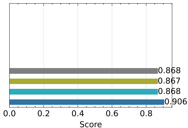
SSIM ↑
