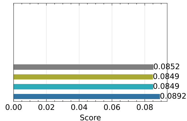
LPIPS ↓
