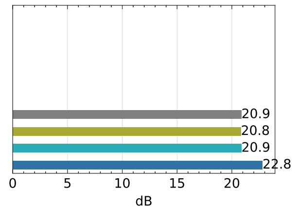
PSNR ↑
