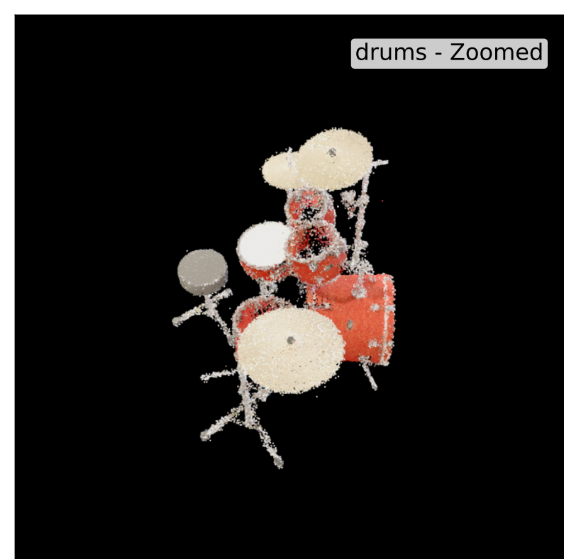
VGGT | | | confidence
