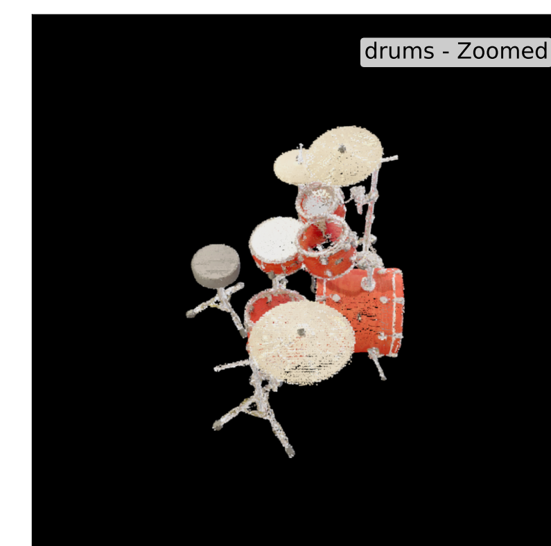
VGGT | | | voxels
