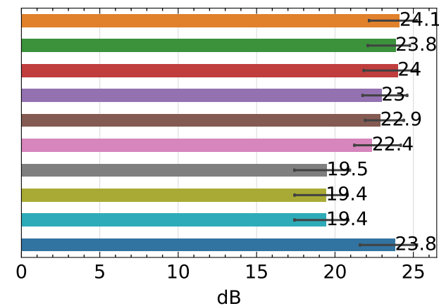
PSNR ↑ - indoor
