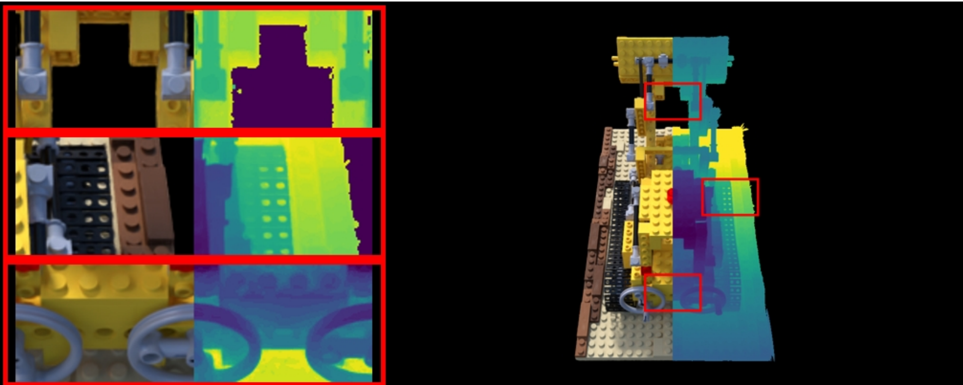
lego: VGGT | 100.0 PSNR: 20.34 | LPIPS: 0.0760 | SSIM: 0.7733
