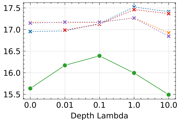
PSNR
