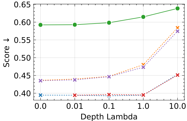
LPIPS
