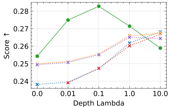
SSIM
