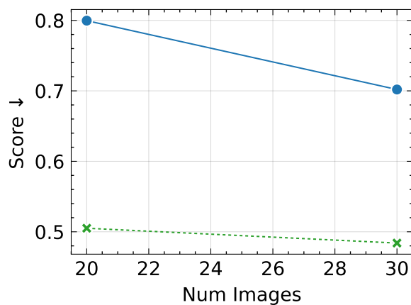
LPIPS
