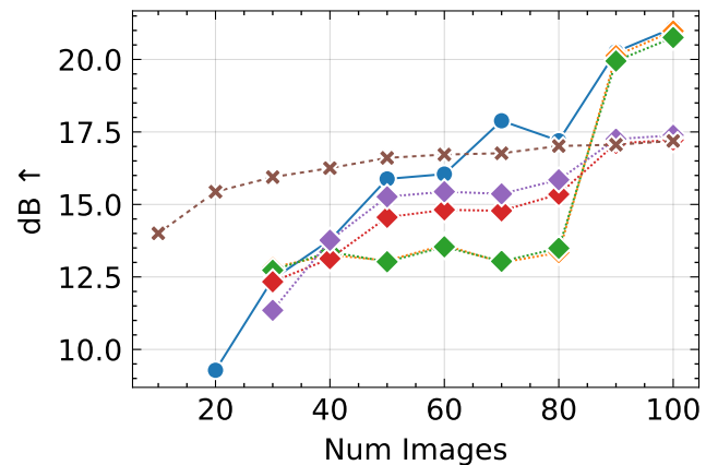
PSNR
