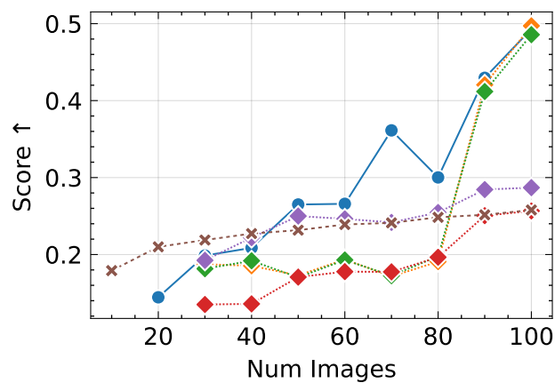
SSIM
