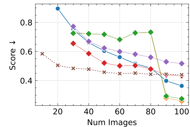
LPIPS
