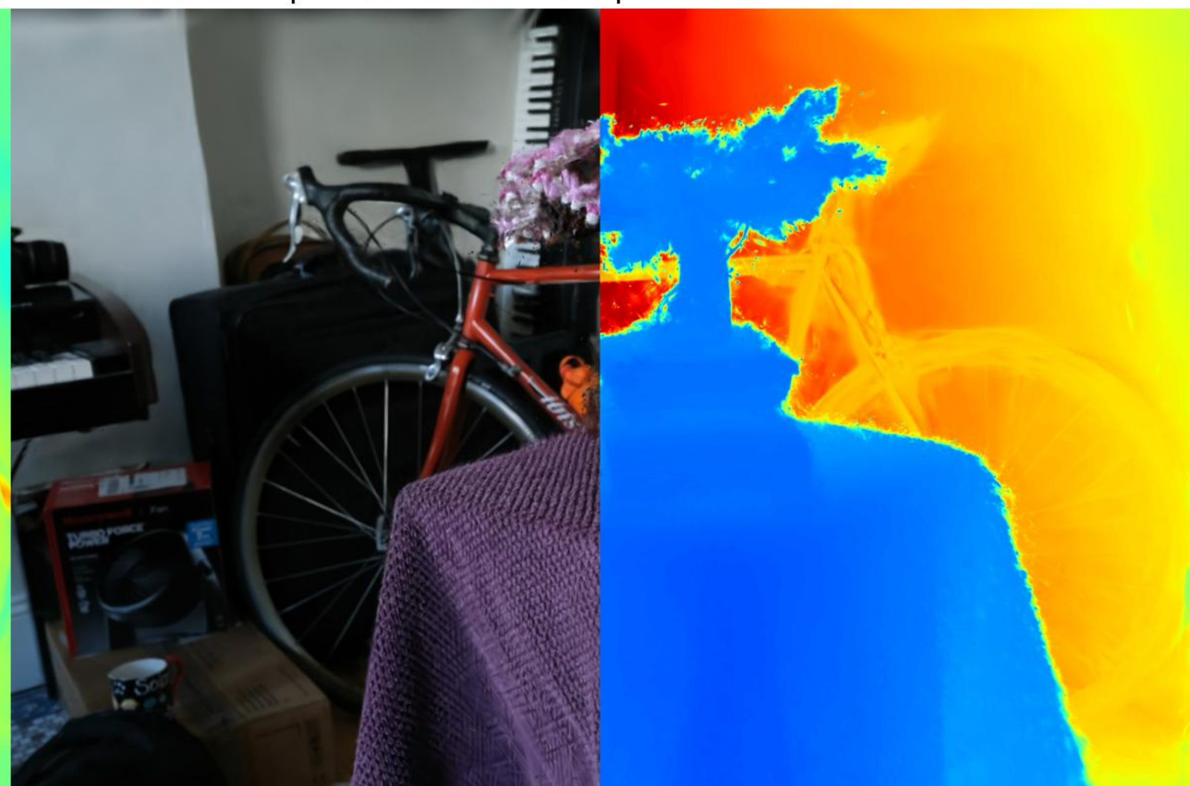
Config: VGGT | | depth_lambda=1.0 PSNR: 17.31 | LPIPS: 0.3396 | SSIM: 0.5638
