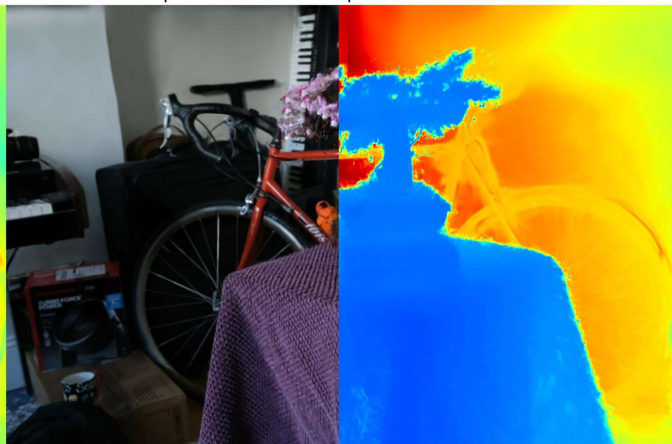
Config: VGGT | standard | depth_lambda=1.0 PSNR: 17.39 | LPIPS: 0.3340 | SSIM: 0.5668
