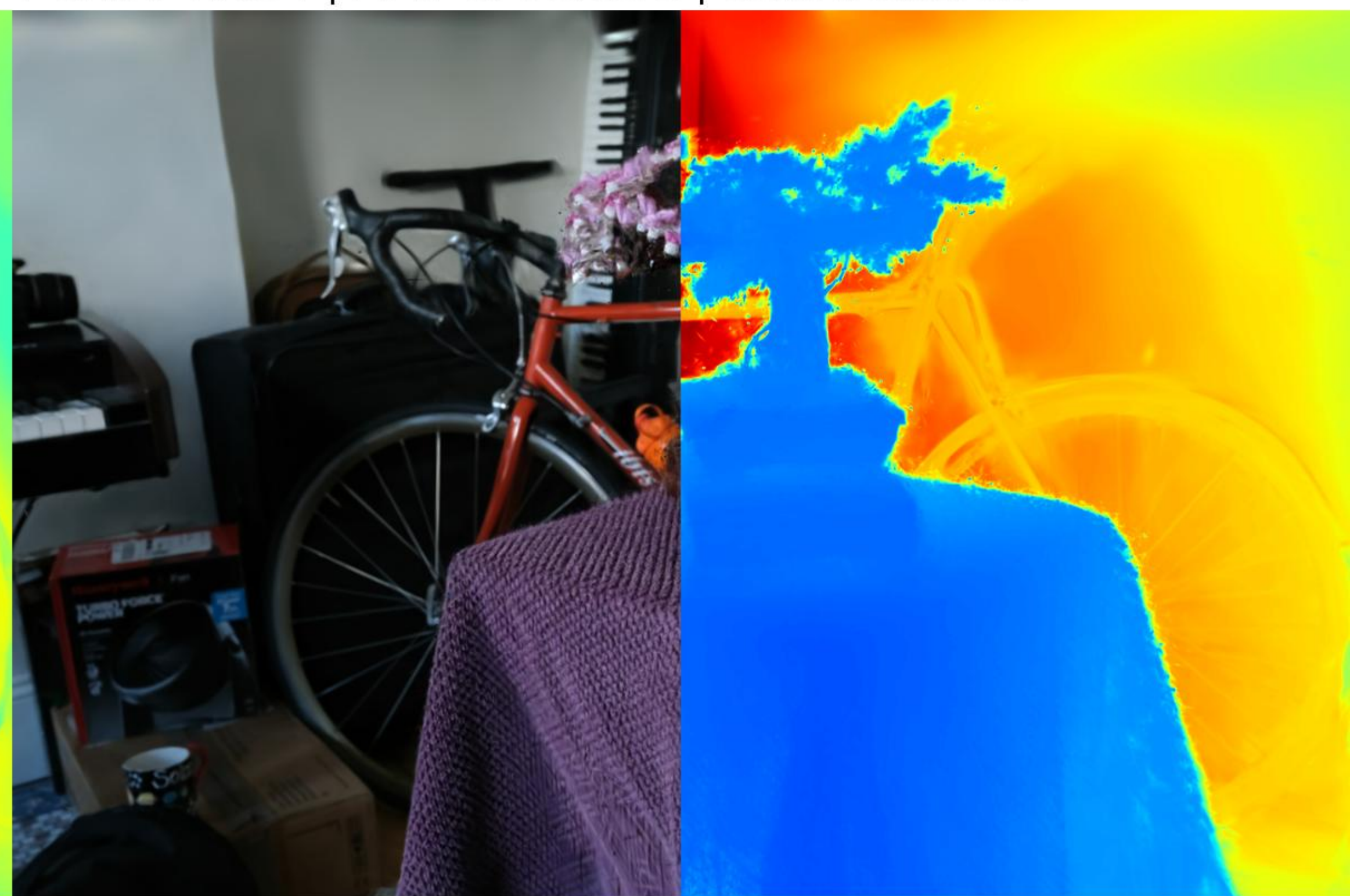
Config: VGGT | sigmoid | depth_lambda=1.0 PSNR: 17.23 | LPIPS: 0.3313 | SSIM: 0.5652
