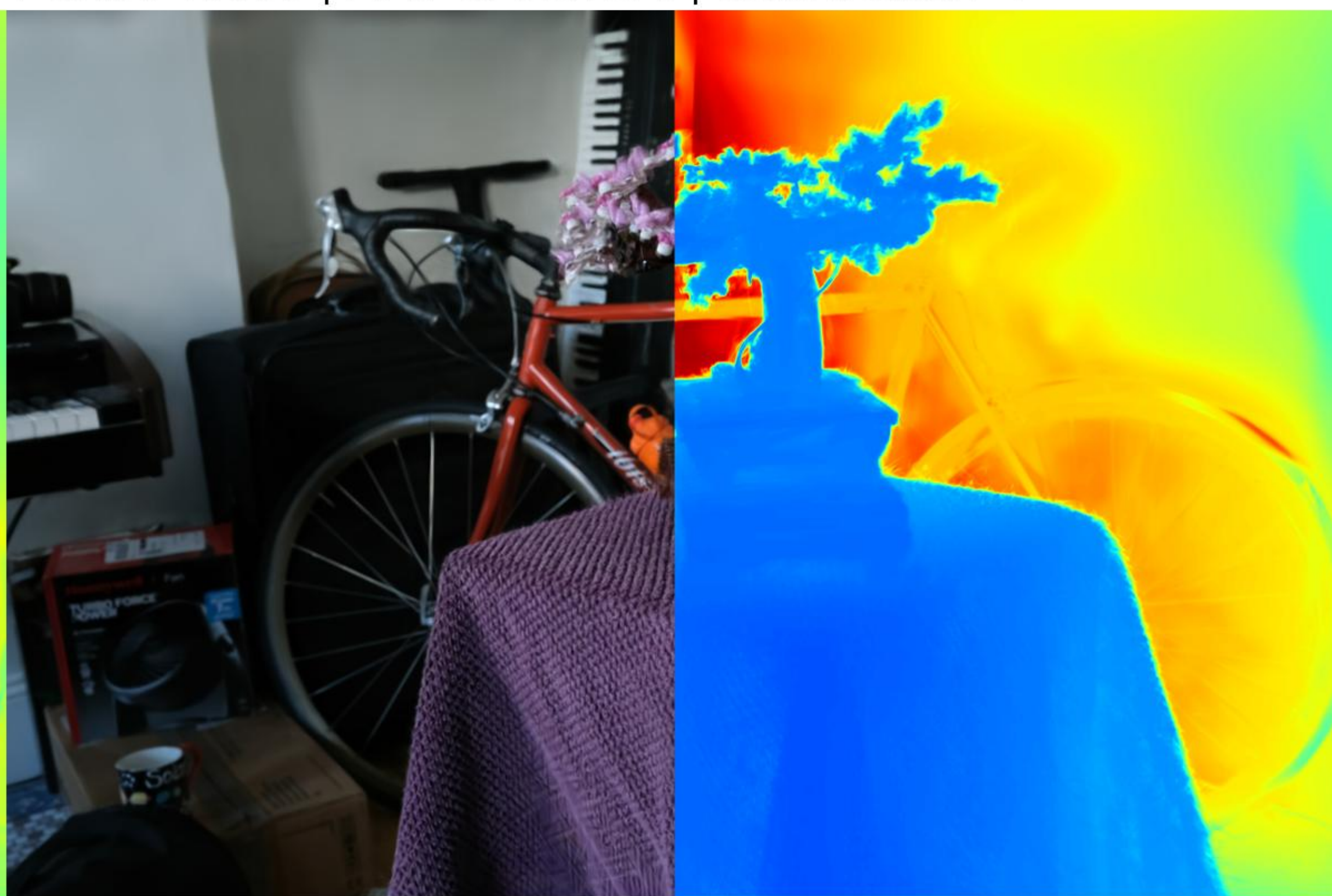
Config: VGGT | sigmoid | depth_lambda=0.01 PSNR: 17.20 | LPIPS: 0.3314 | SSIM: 0.5700
