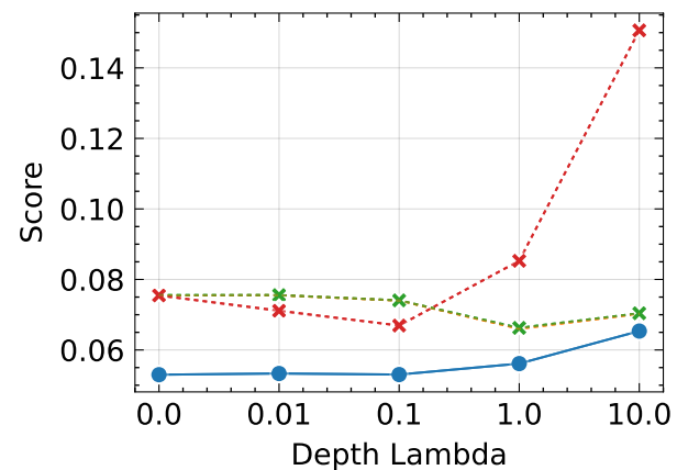
LPIPS ↓
