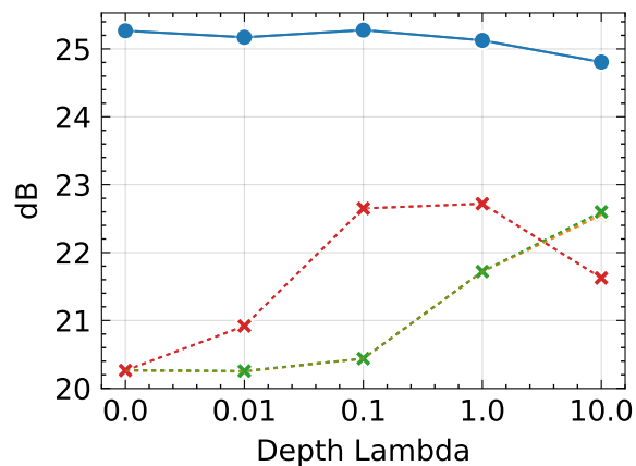
PSNR ↑
