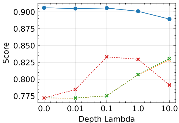
SSIM ↑
