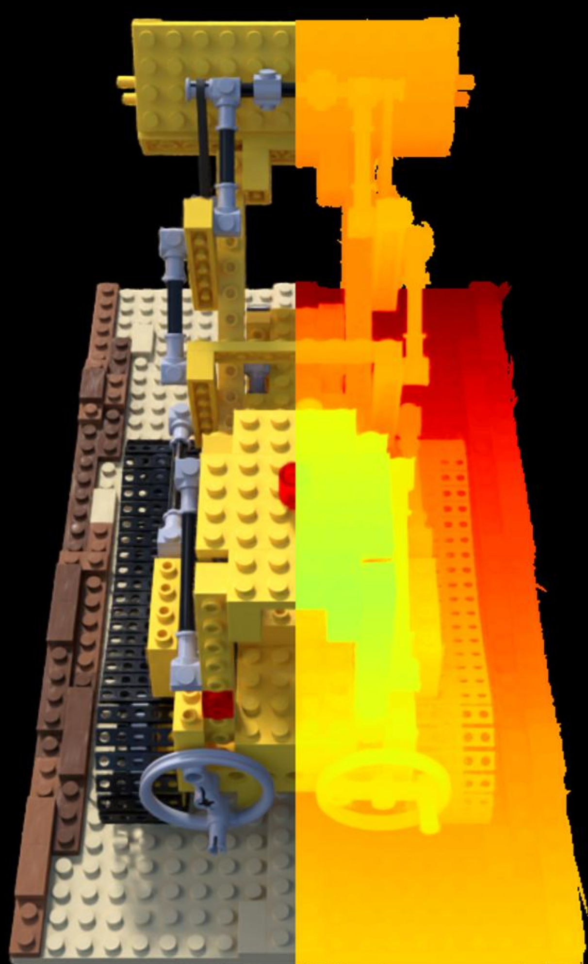
Config: VGGT | standard | depth_lambda=0.0 PSNR: 24.52 | LPIPS: 0.0524 | SSIM: 0.8957
