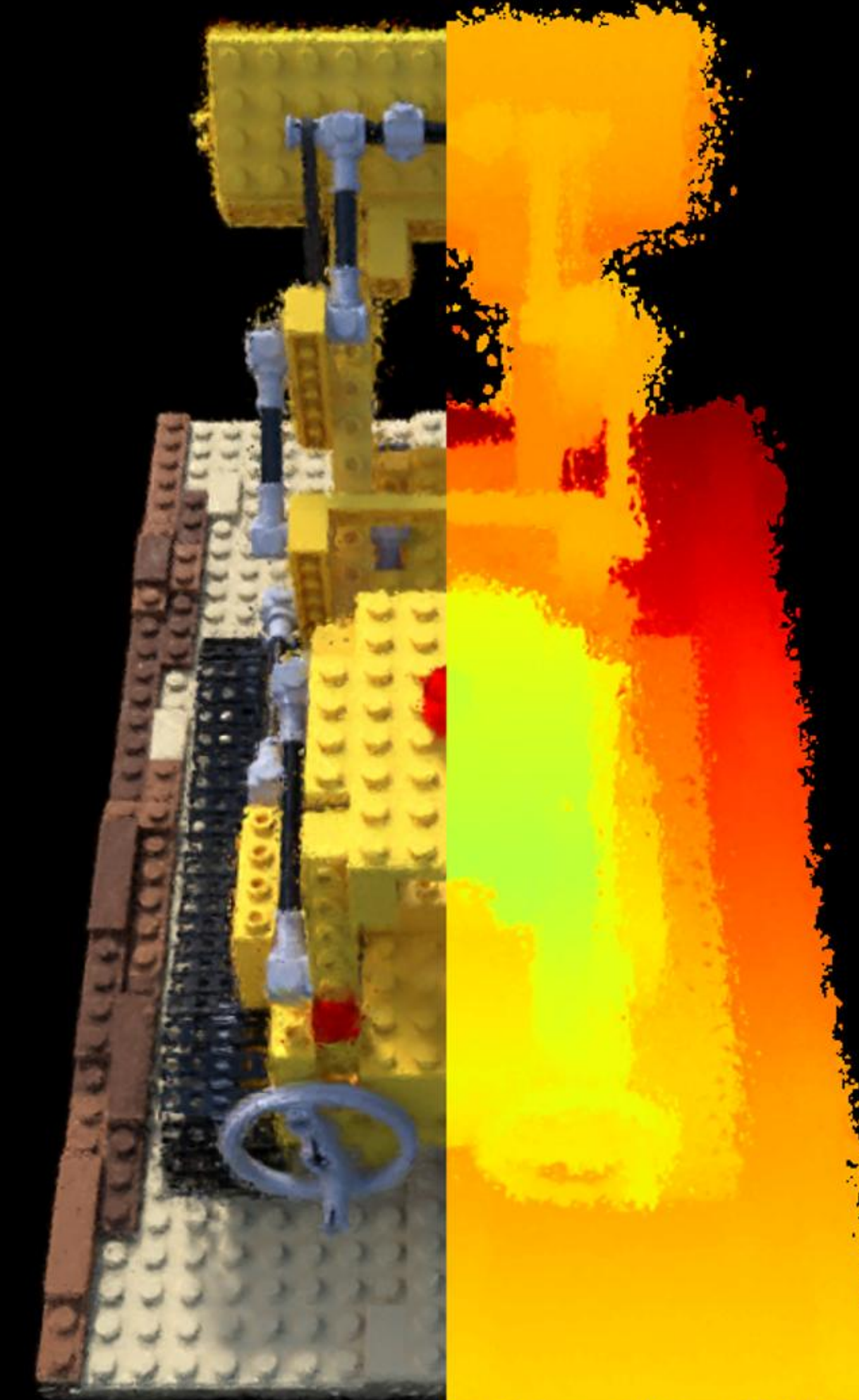
Config: VGGT | standard | depth_lambda=1.0 PSNR: 22.92 | LPIPS: 0.0986 | SSIM: 0.8337
