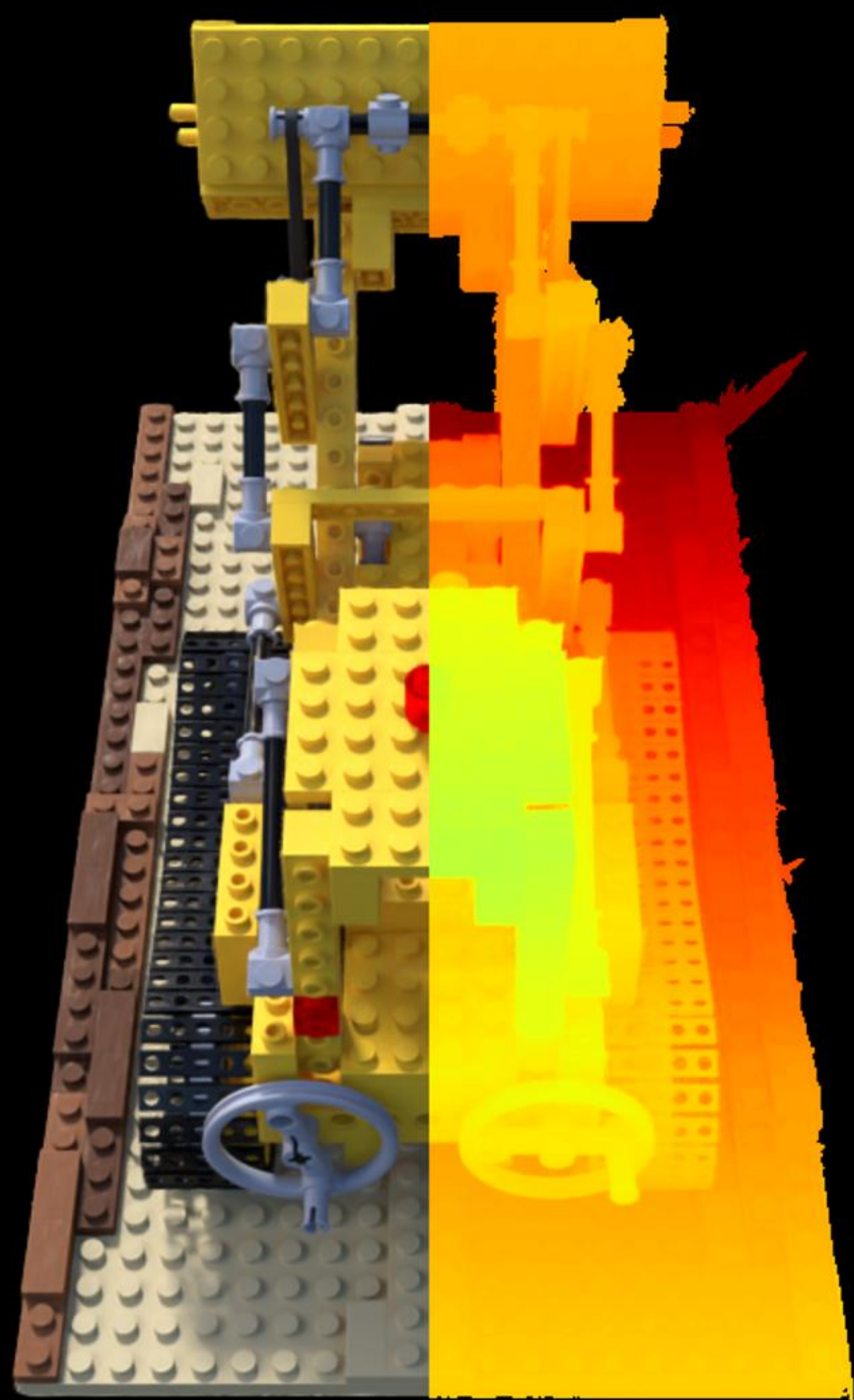
Config: VGGT | | depth_lambda=0.0 PSNR: 24.55 | LPIPS: 0.0527 | SSIM: 0.8962
