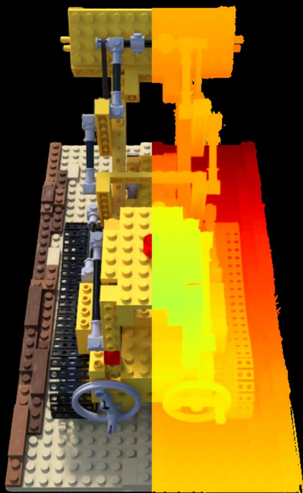
Config: VGGT | | depth_lambda=0.01 PSNR: 24.44 | LPIPS: 0.0533 | SSIM: 0.8929
