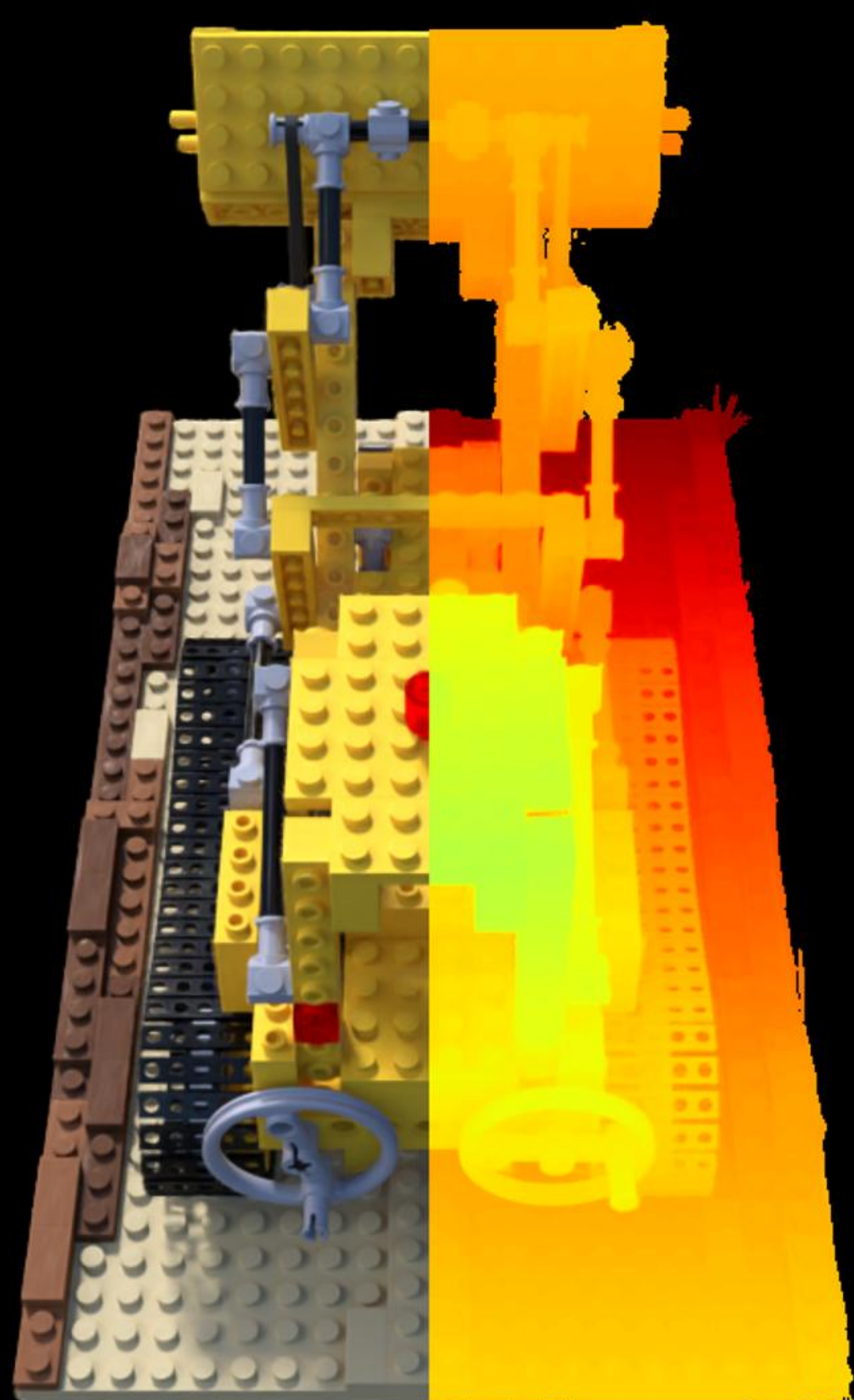
Config: VGGT | sigmoid | depth_lambda=0.0 PSNR: 24.54 | LPIPS: 0.0531 | SSIM: 0.8961
