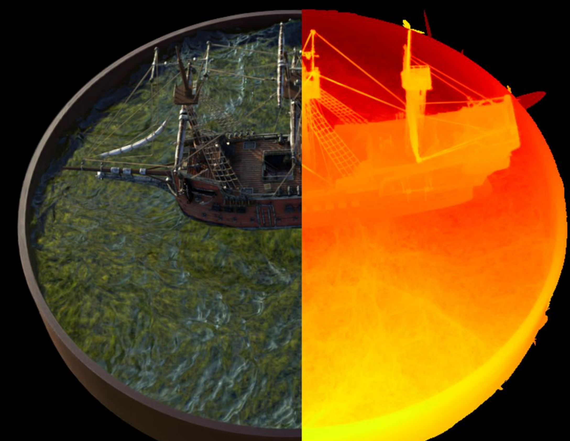
Config: VGGT | sigmoid | depth_lambda=0.0 PSNR: 23.93 | LPIPS: 0.1553 | SSIM: 0.6651
