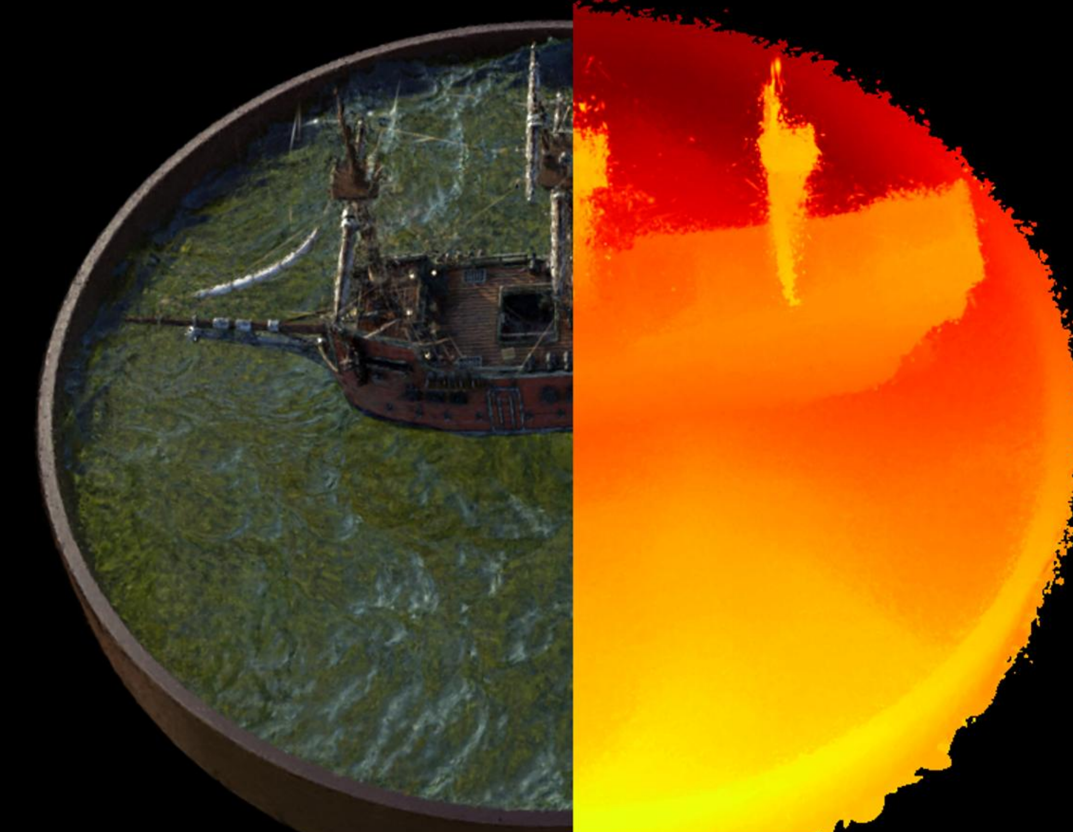
Config: VGGT | standard | depth_lambda=1.0 PSNR: 23.20 | LPIPS: 0.1675 | SSIM: 0.6455
