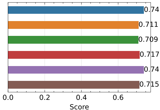
SSIM ↑
