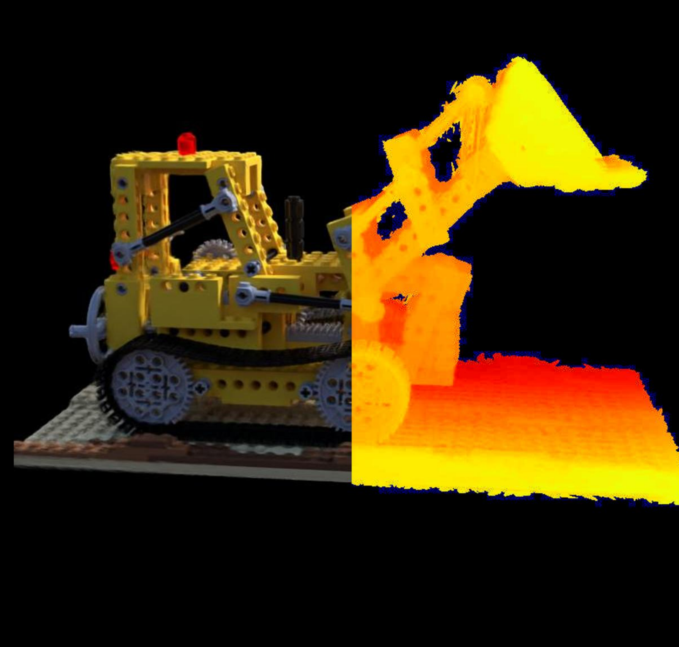
Config: VGGT | PSNR: 16.27 | LPIPS: 0.2734 | SSIM: 0.6864
