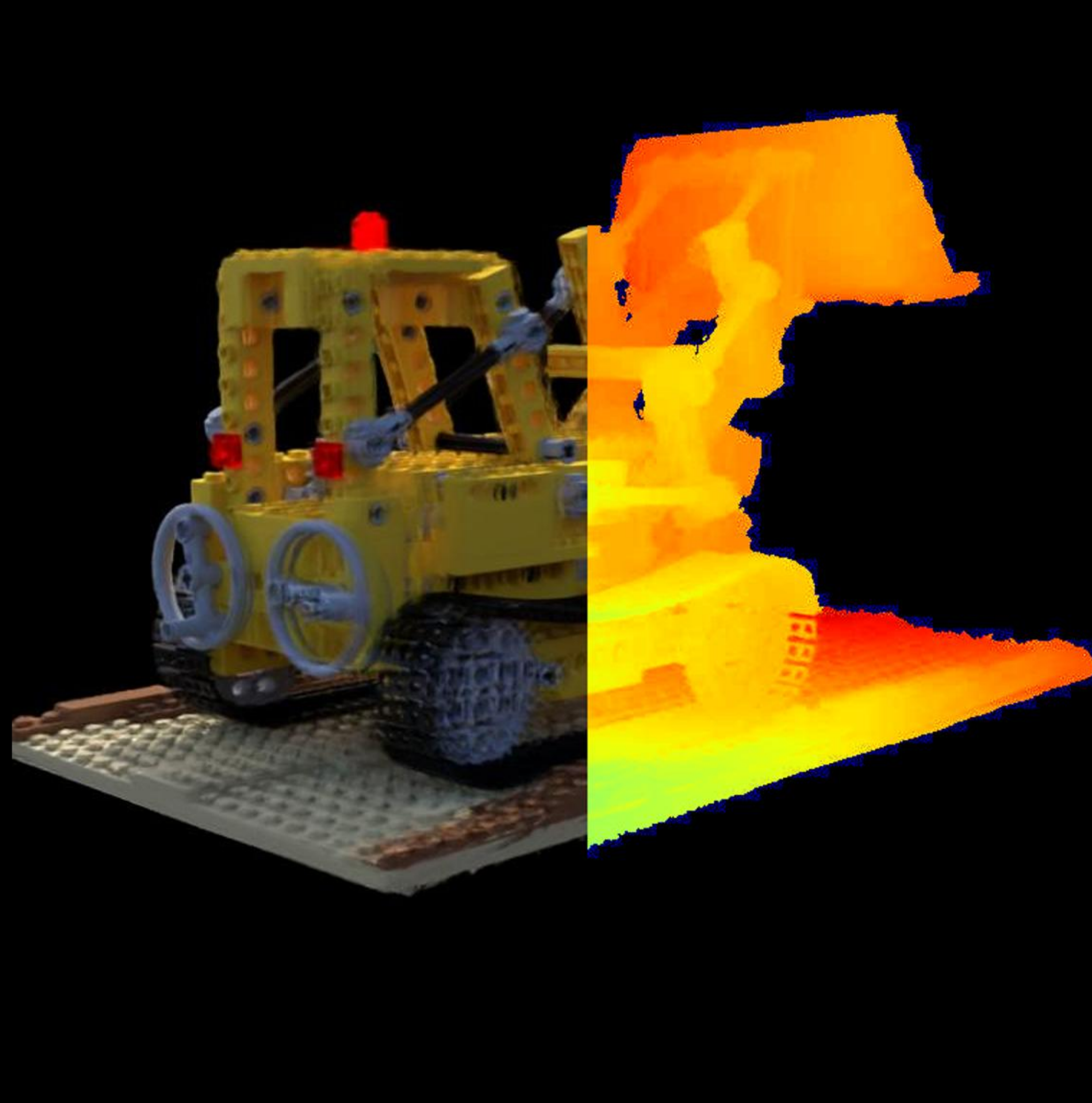
Config: VGGT | sigmoid PSNR: 17.56 | LPIPS: 0.2483 | SSIM: 0.7135
