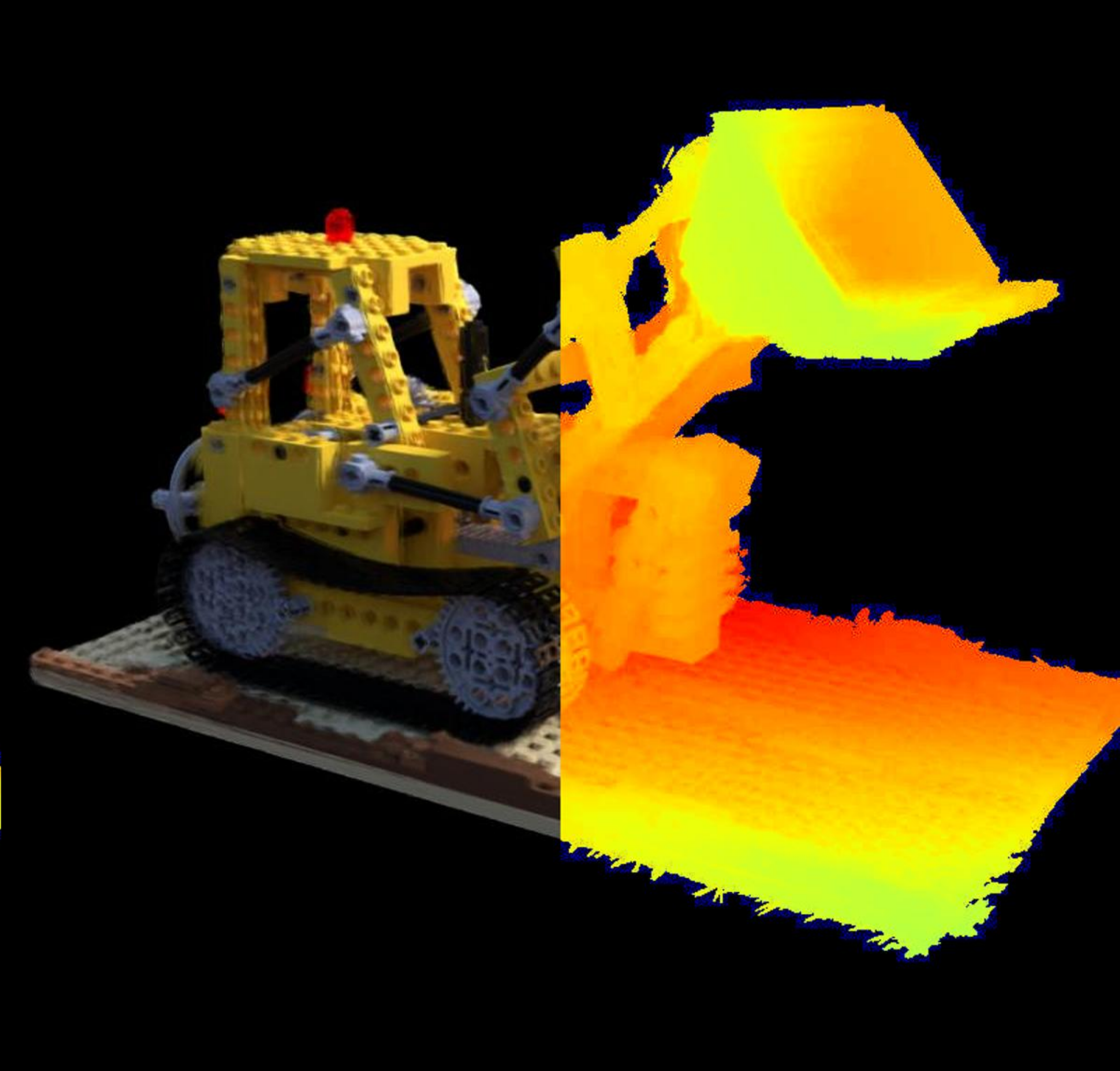
Config: VGGT | PSNR: 14.49 | LPIPS: 0.2962 | SSIM: 0.6648
