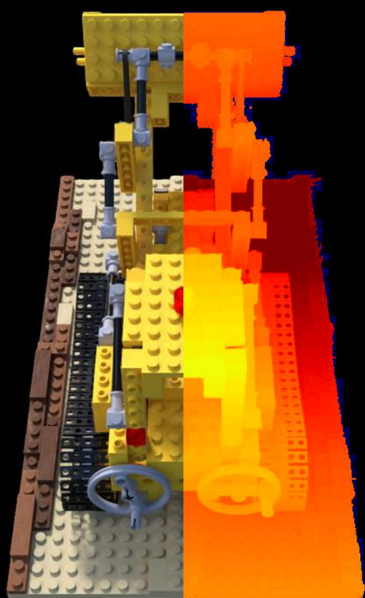
Config: VGGT | | depth_lambda=0.0 PSNR: 26.04 | LPIPS: 0.0445 | SSIM: 0.9341
