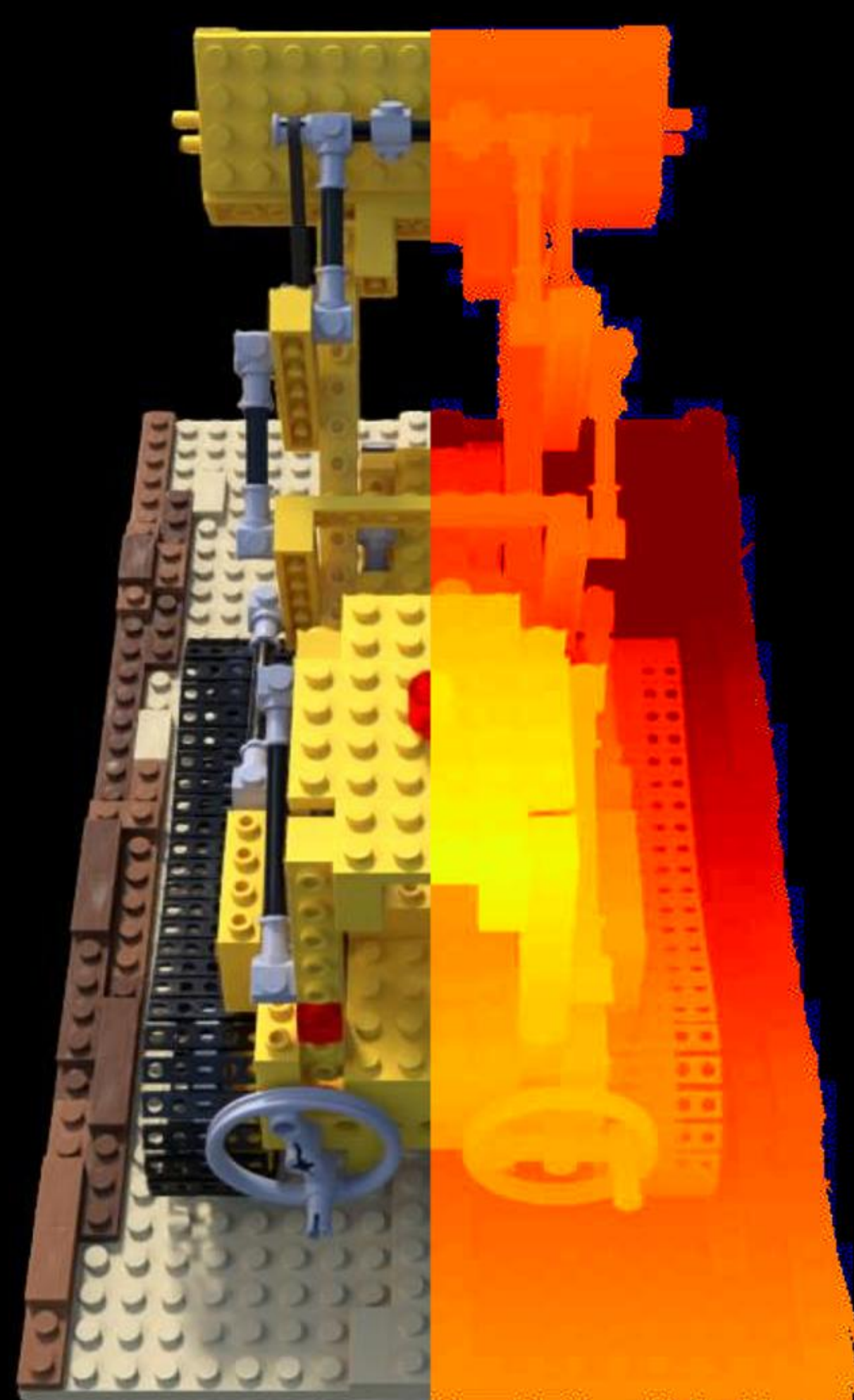
Config: VGGT | | depth_lambda=0.01 PSNR: 26.04 | LPIPS: 0.0450 | SSIM: 0.9337
