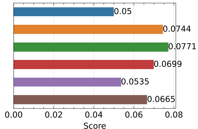
LPIPS ↓
