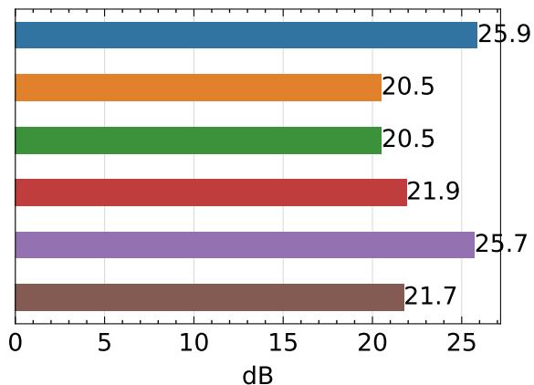
PSNR ↑
