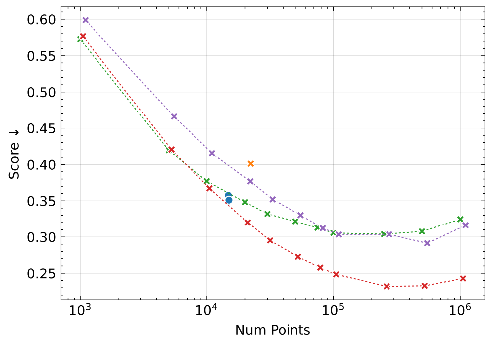
LPIPS
