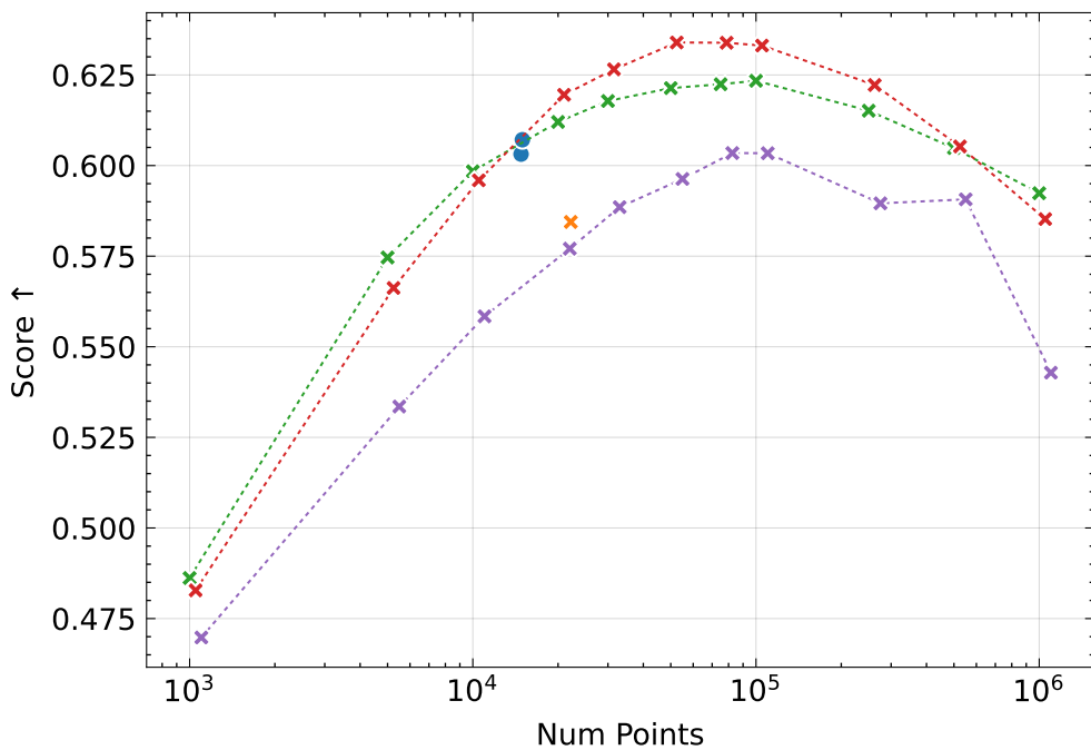
SSIM
