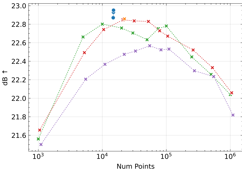
PSNR
